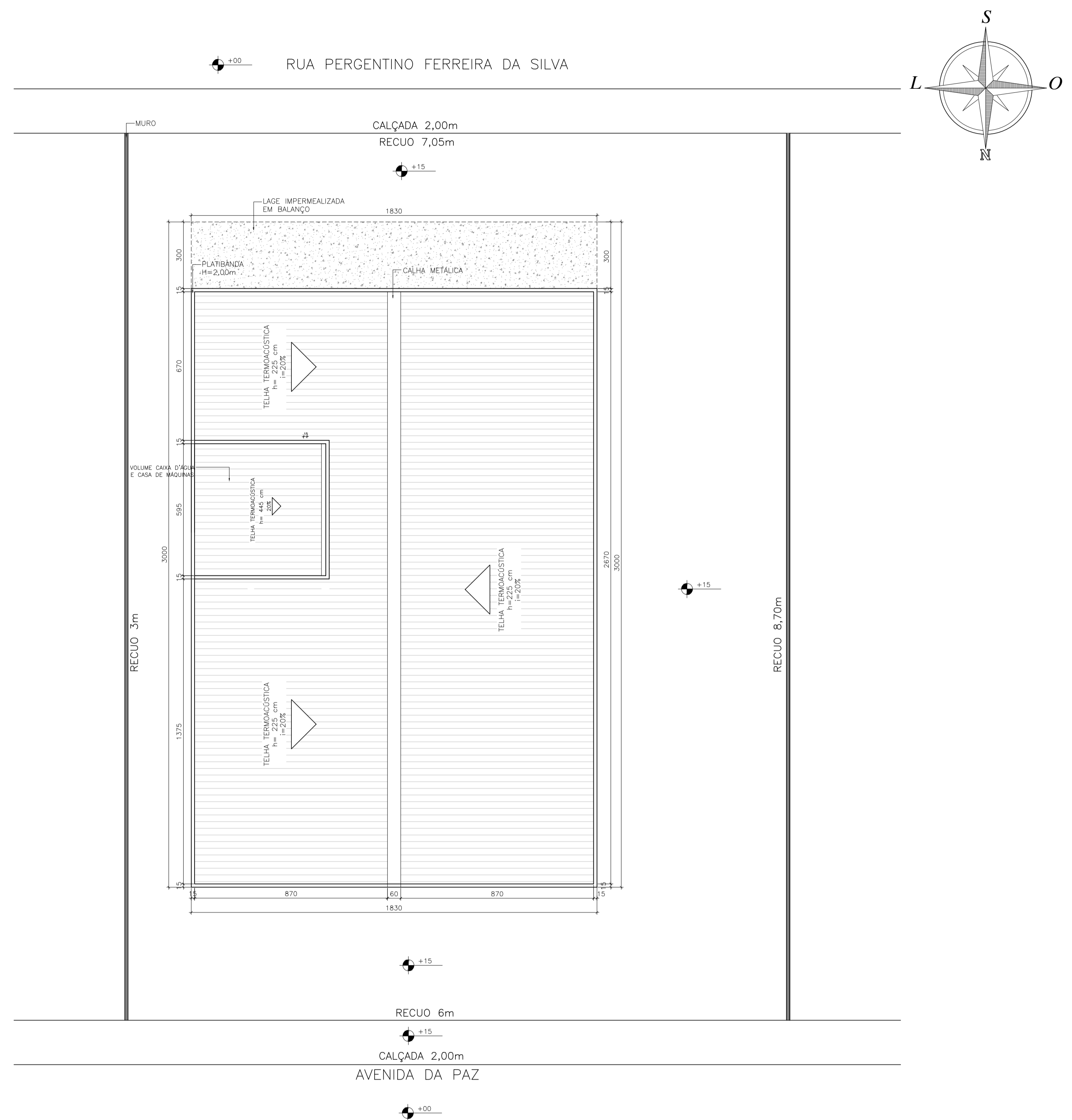
02 PLANTA COBERTURA ESCALA 1:125 ESCALA GRÁFICA
