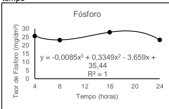
Gráfico 14: Teor de fósforo em relação ao tempo
