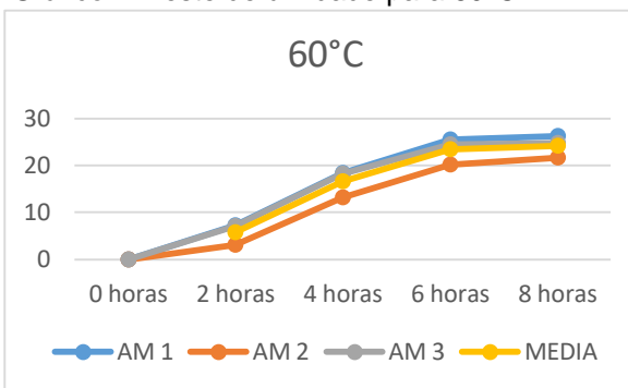
Gráfico 2: Teste de umidade para 60°C
