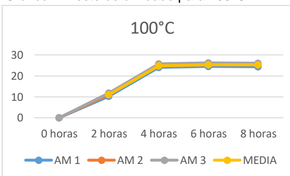
Gráfico 4: Teste de umidade para 100°C
