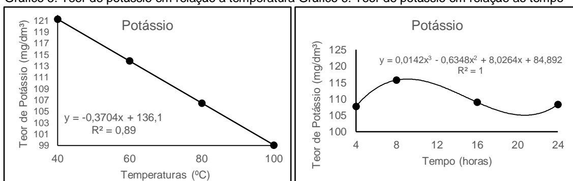
Gráfico 5: Teor de potássio em relação a temperatura Gráfico 6: Teor de potássio em relação ao tempo
