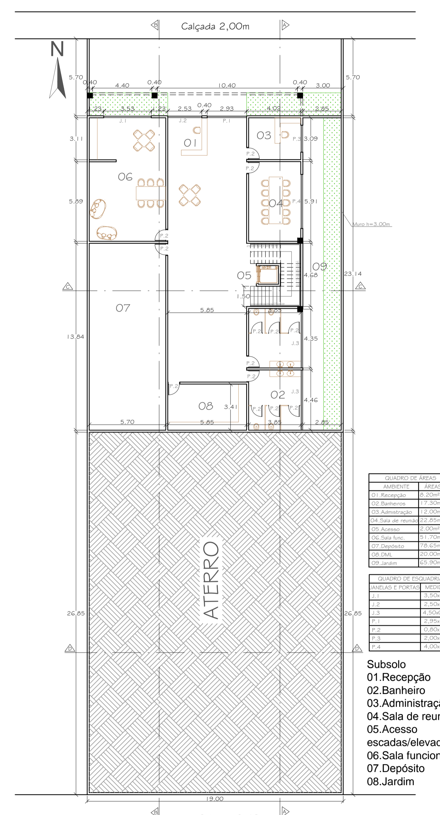
PLANTA SUBSOLO
