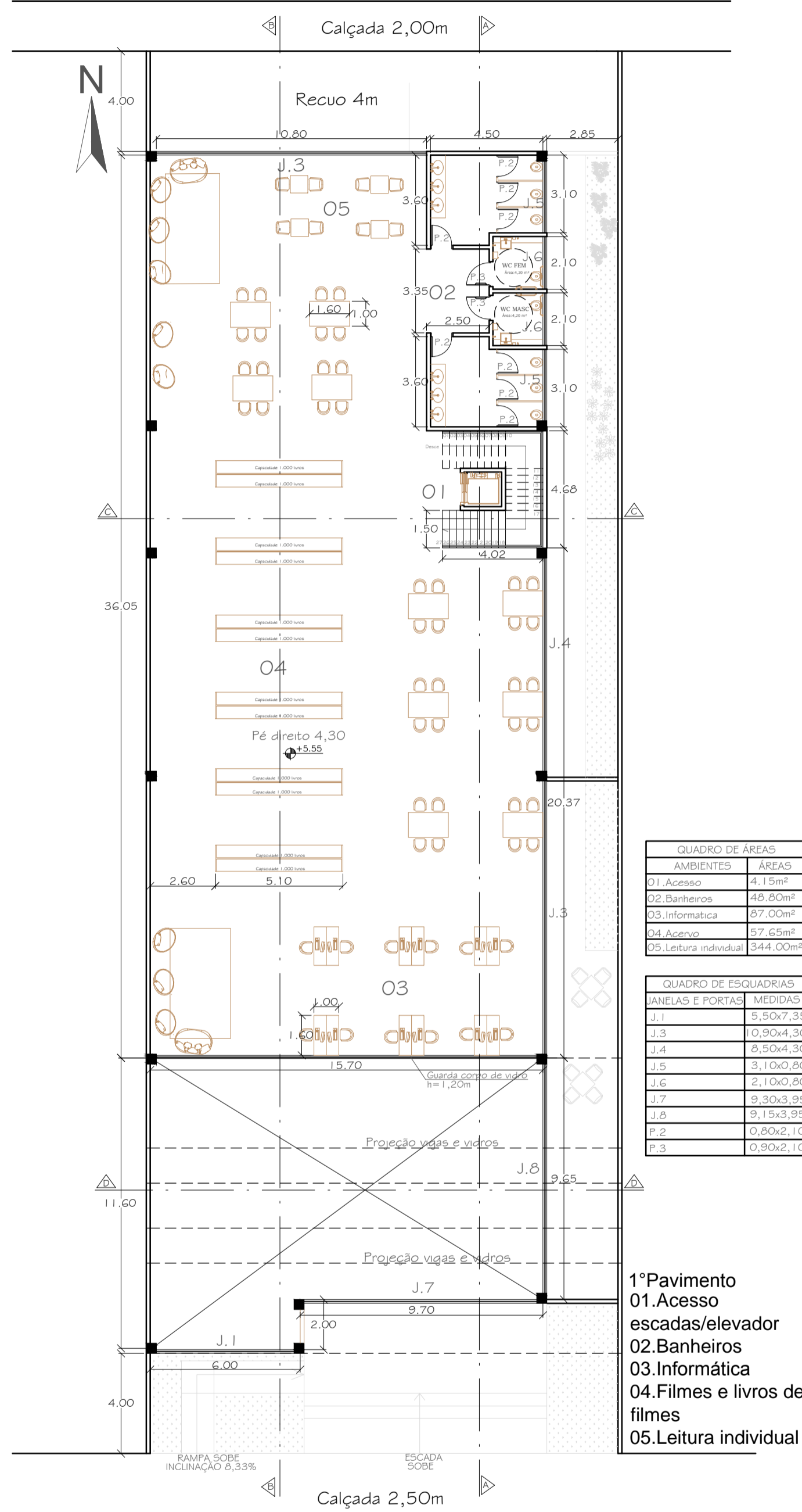
PLANTA 1º PAVTO
