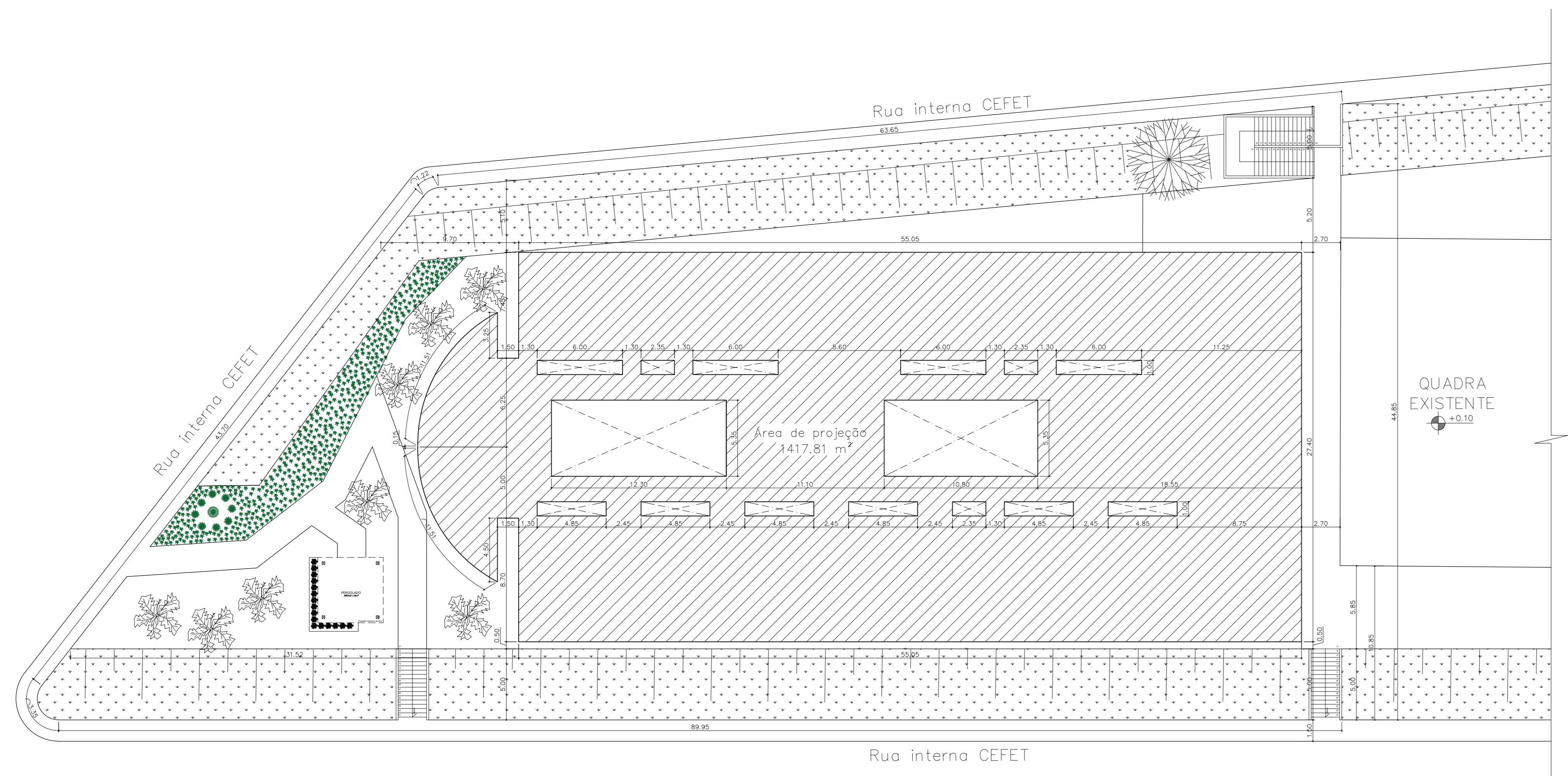
IMPLANTAÇÃO Escala 1/200
