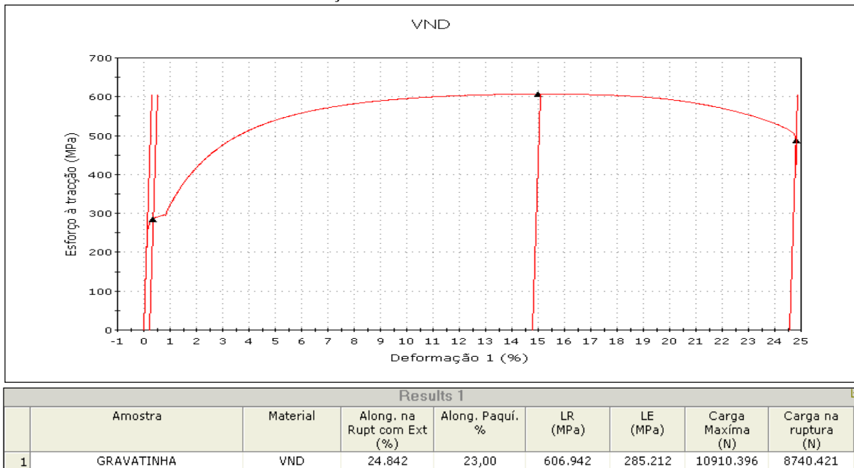
Gráfico 1 - Gráfico de curva de tensão do aço VND
