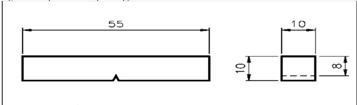
Figura 4 - Corpo de Prova Tipo Charpy
