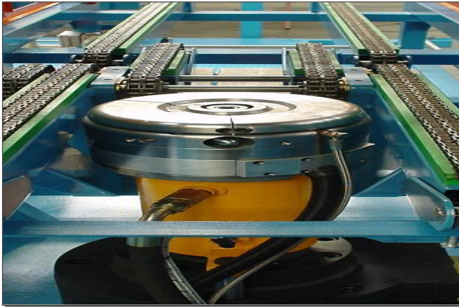
Figura 1 - Prensa de puncionar
