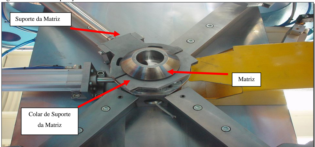
Figura 2 - Matriz em posição de corte
