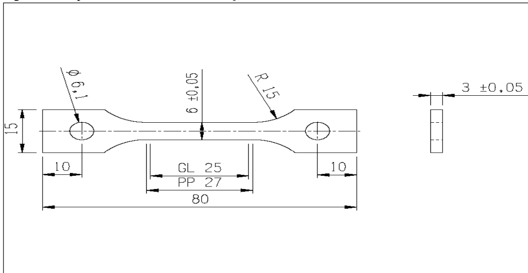
Figura 3 - Corpo de Prova de Ensaio de Tração
