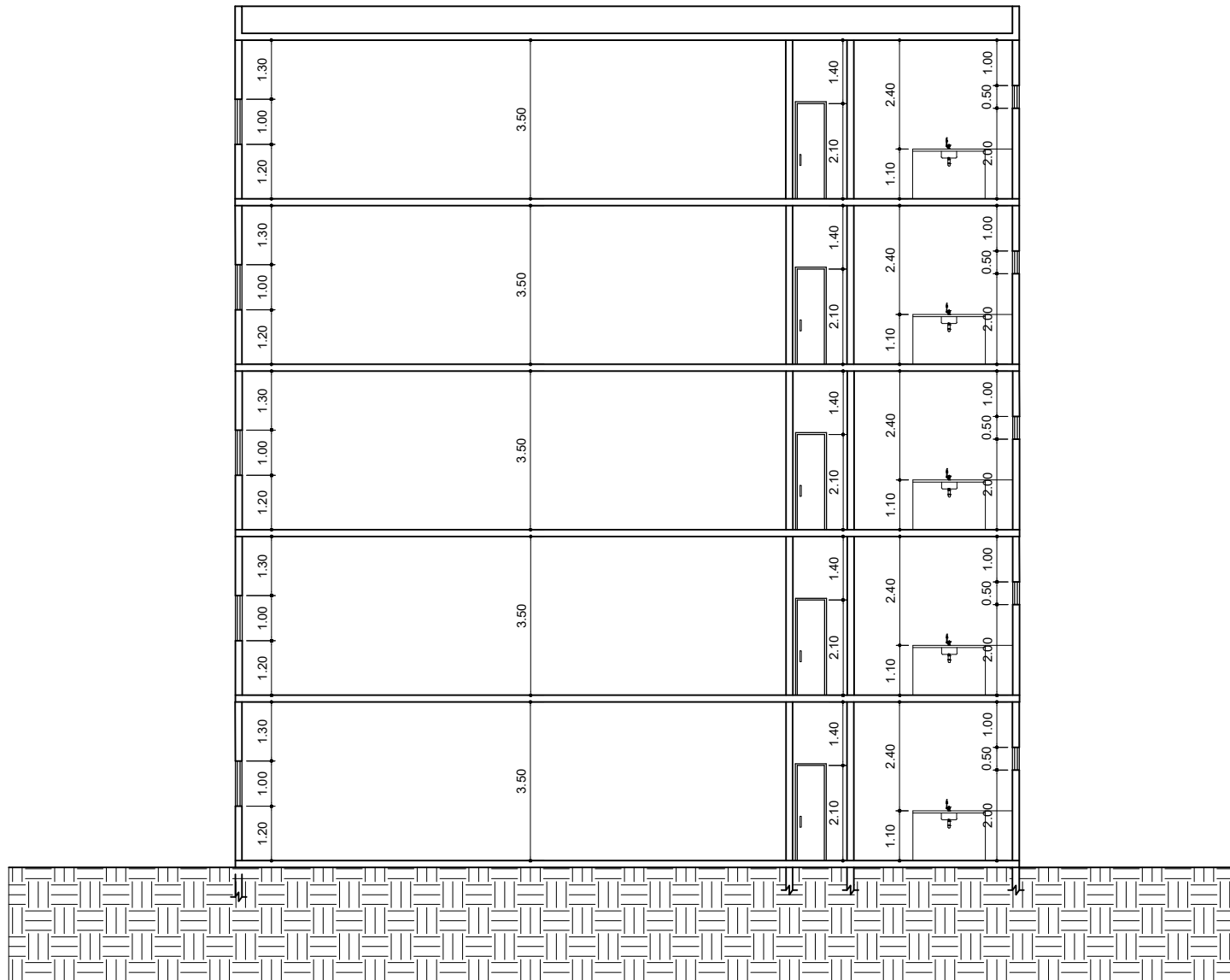
FIGURA 03 - CORTE CD ESCALA 1/100
