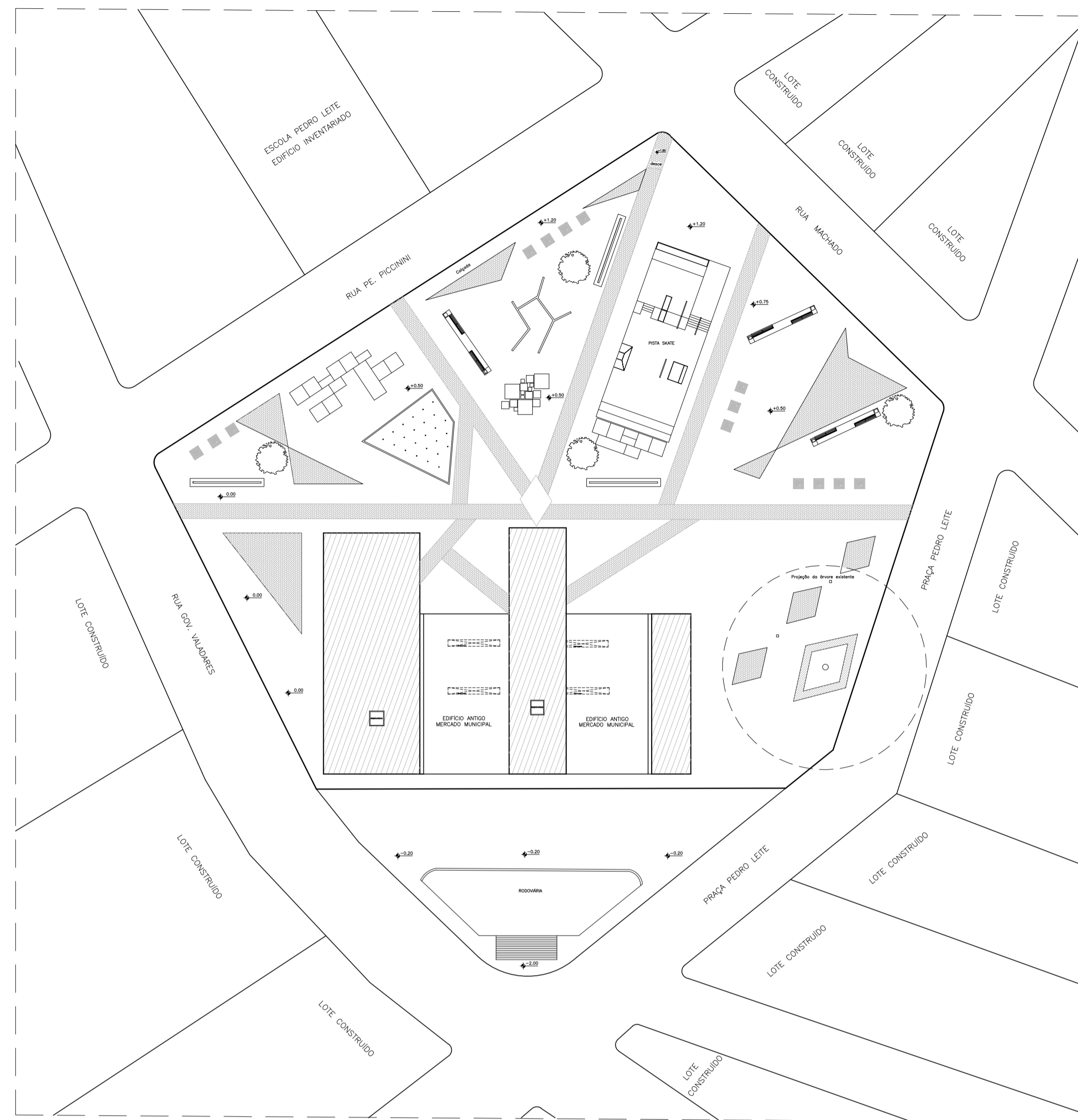
PLANTA DE SITUAÇÃO ESC: 1/500
