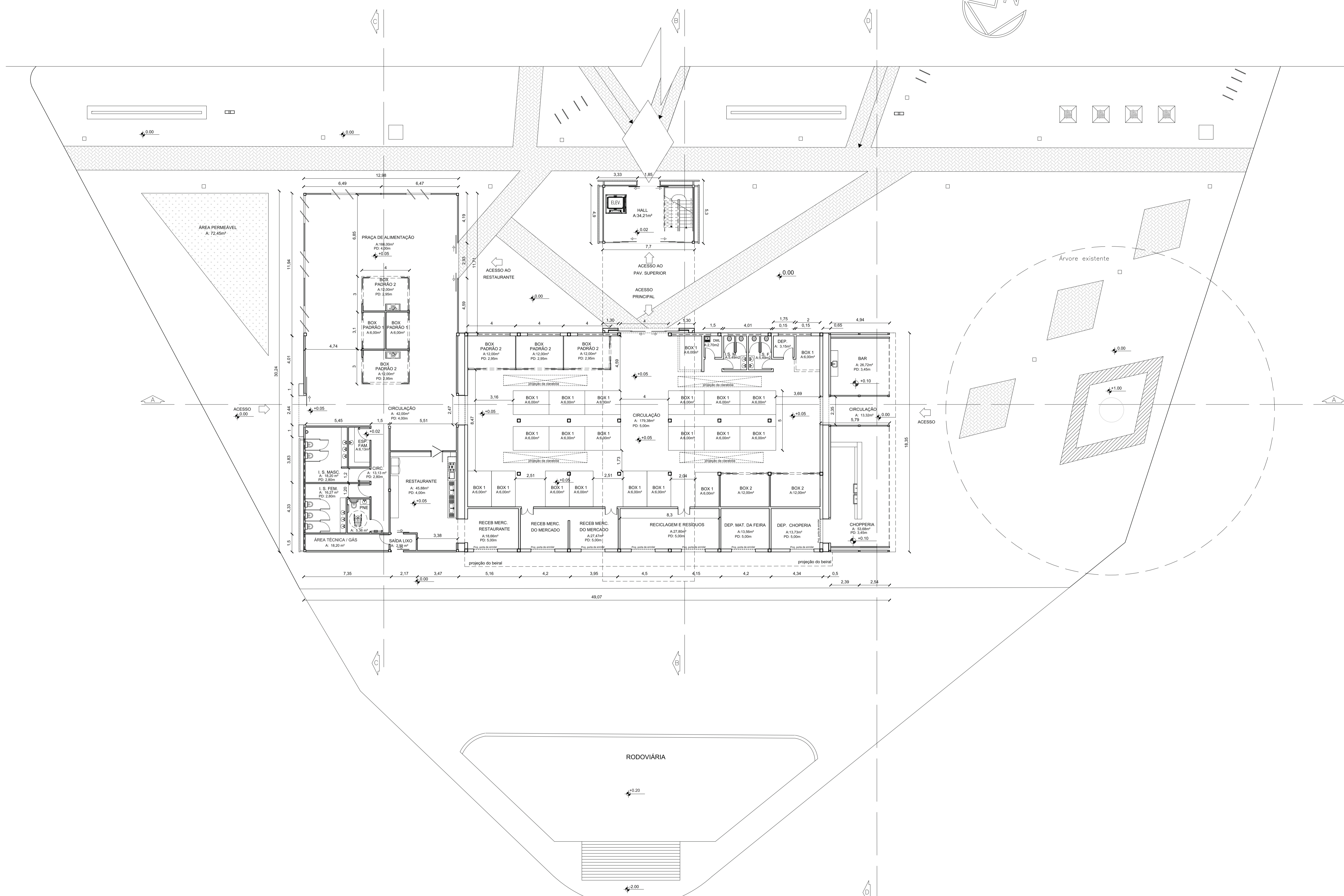
PLANTA PAVIMENTO TÉRREO ESC: 1/150
