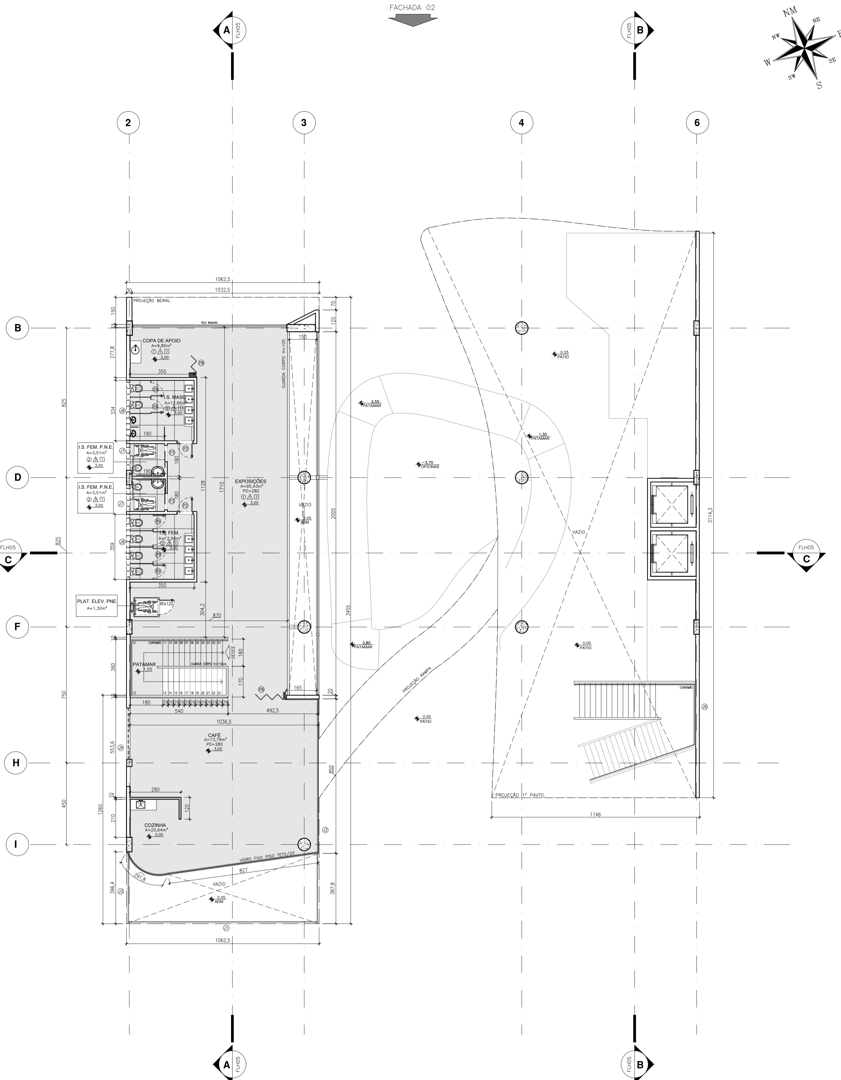
07 PLANTA 1º PAVIMENTO esc: 1:125 A=392m²
