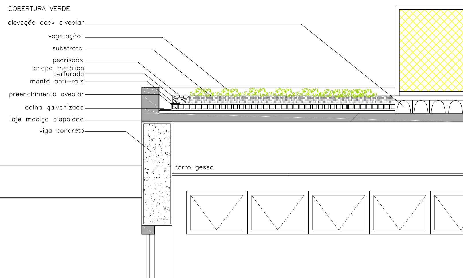
△ DETALHE COBERTURA VERDE escala 1:25
