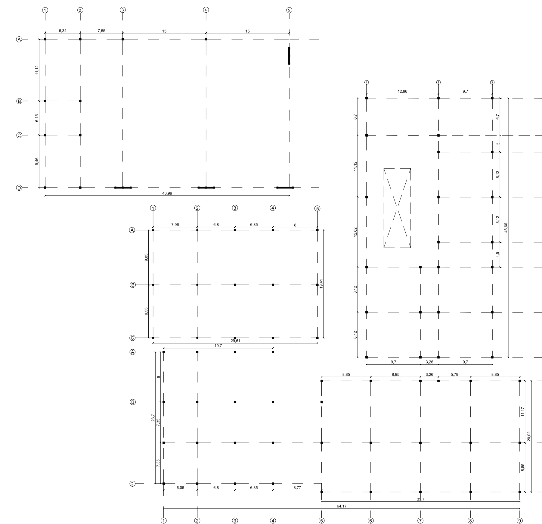
DIAGRAMA ESTRUTURAL Esc.: 1/300
