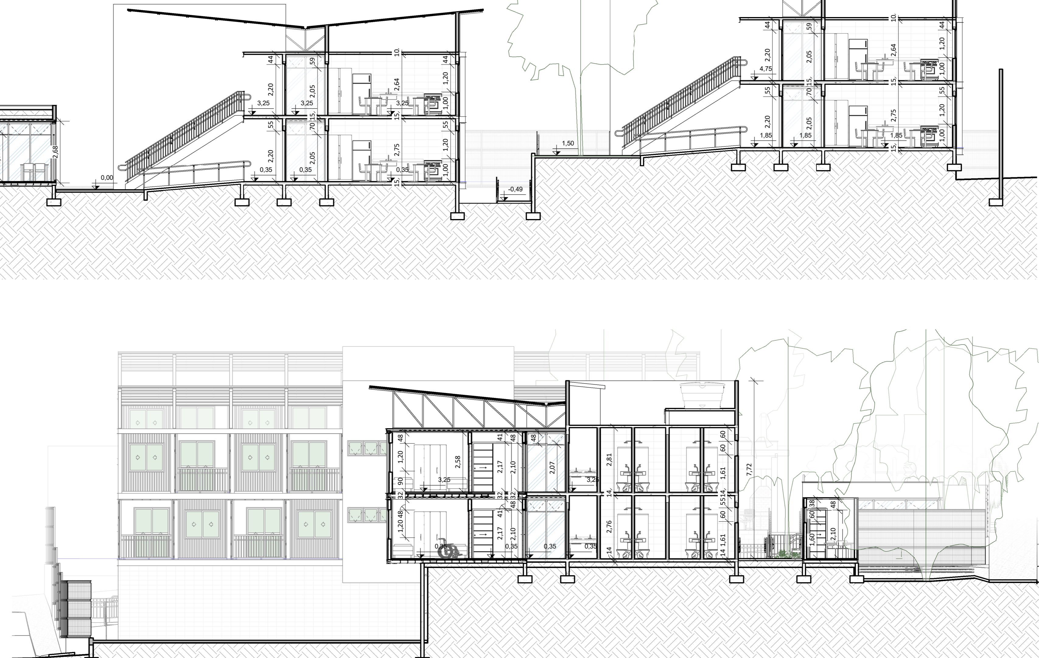
4 C 1:100
