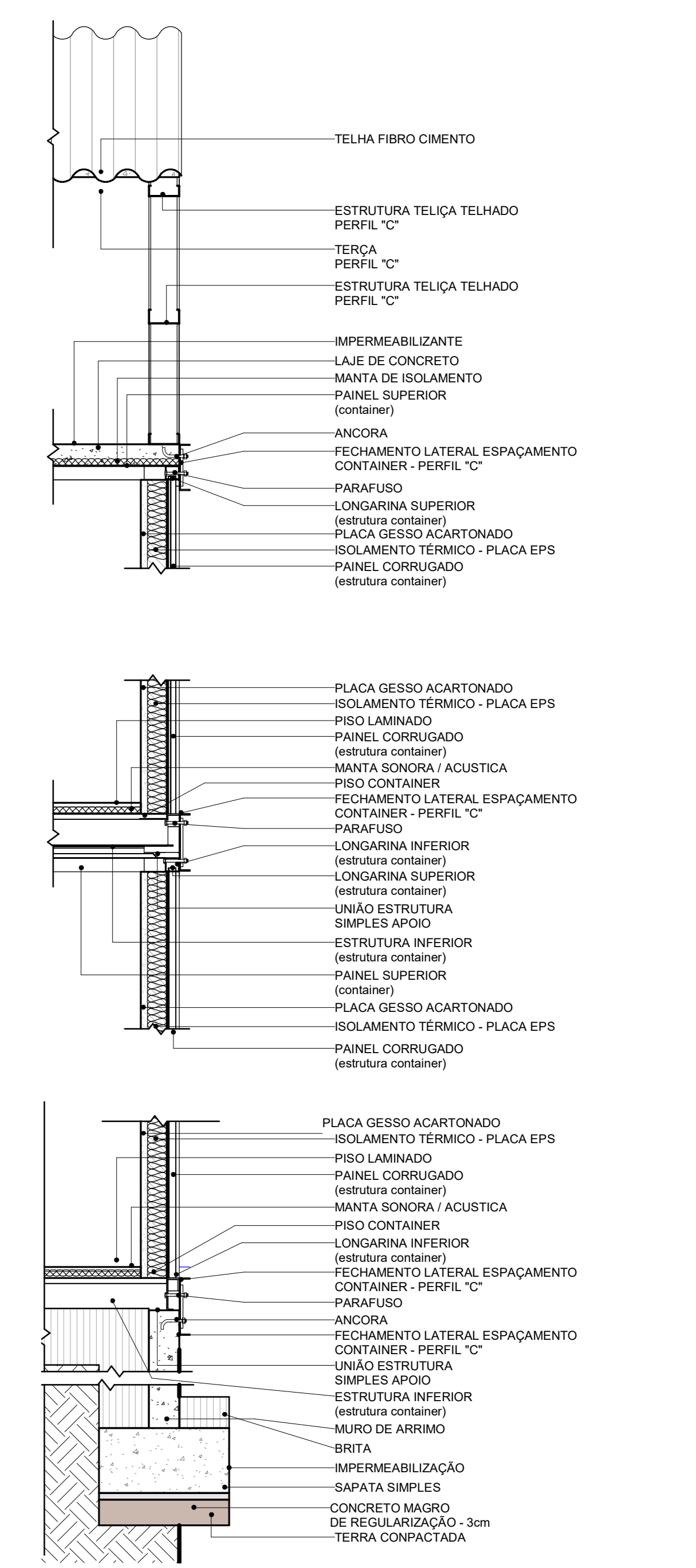
5 DETALHE - 1:20
