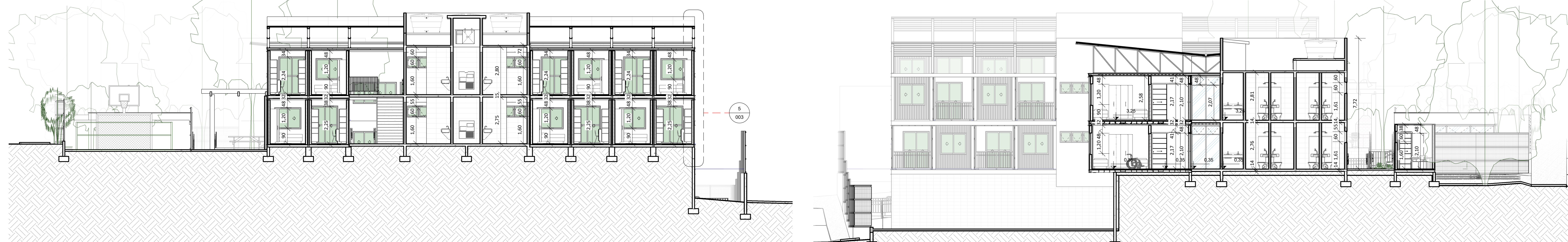
3 B 1:100
