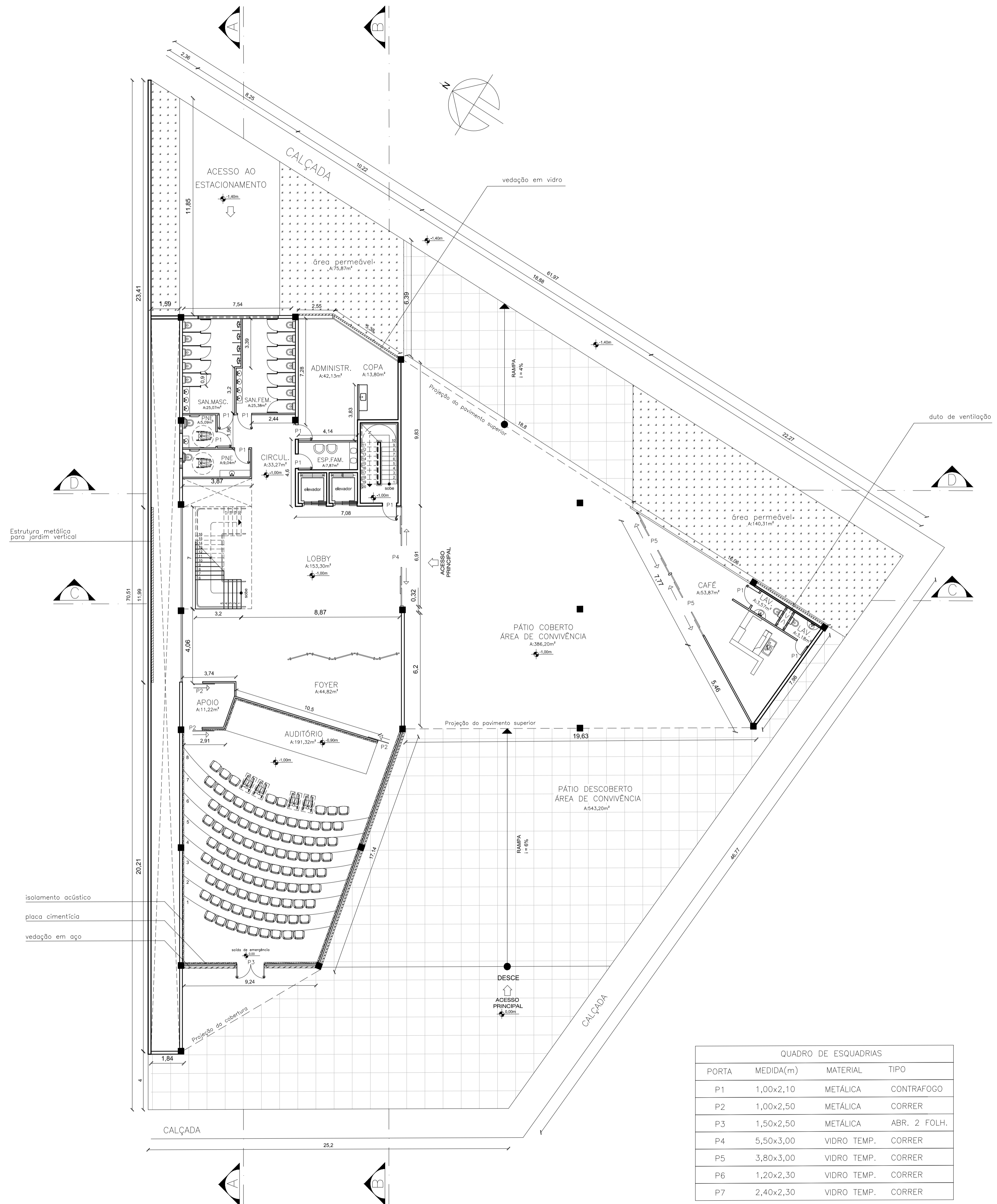
PLANTA PAVIMENTO TÉRREO ESC: 1/125
