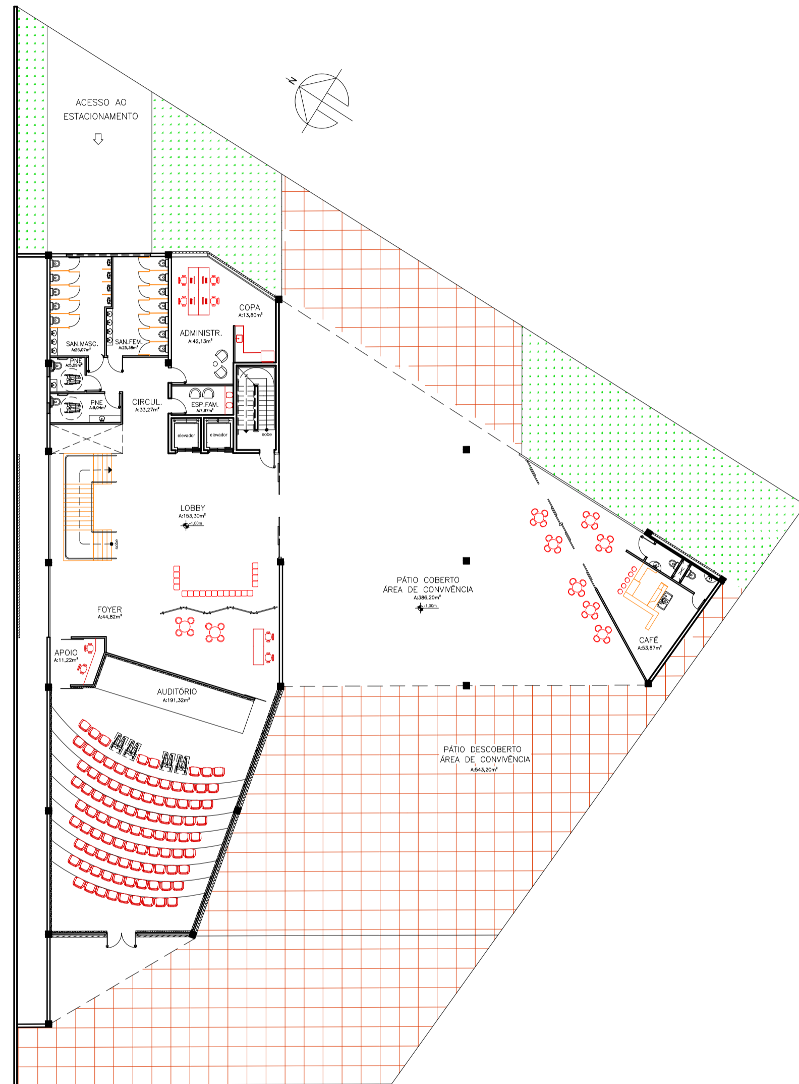
PLANTA PAVIMENTO TÉRREO (HUMANIZADA) ESC: 1/200
