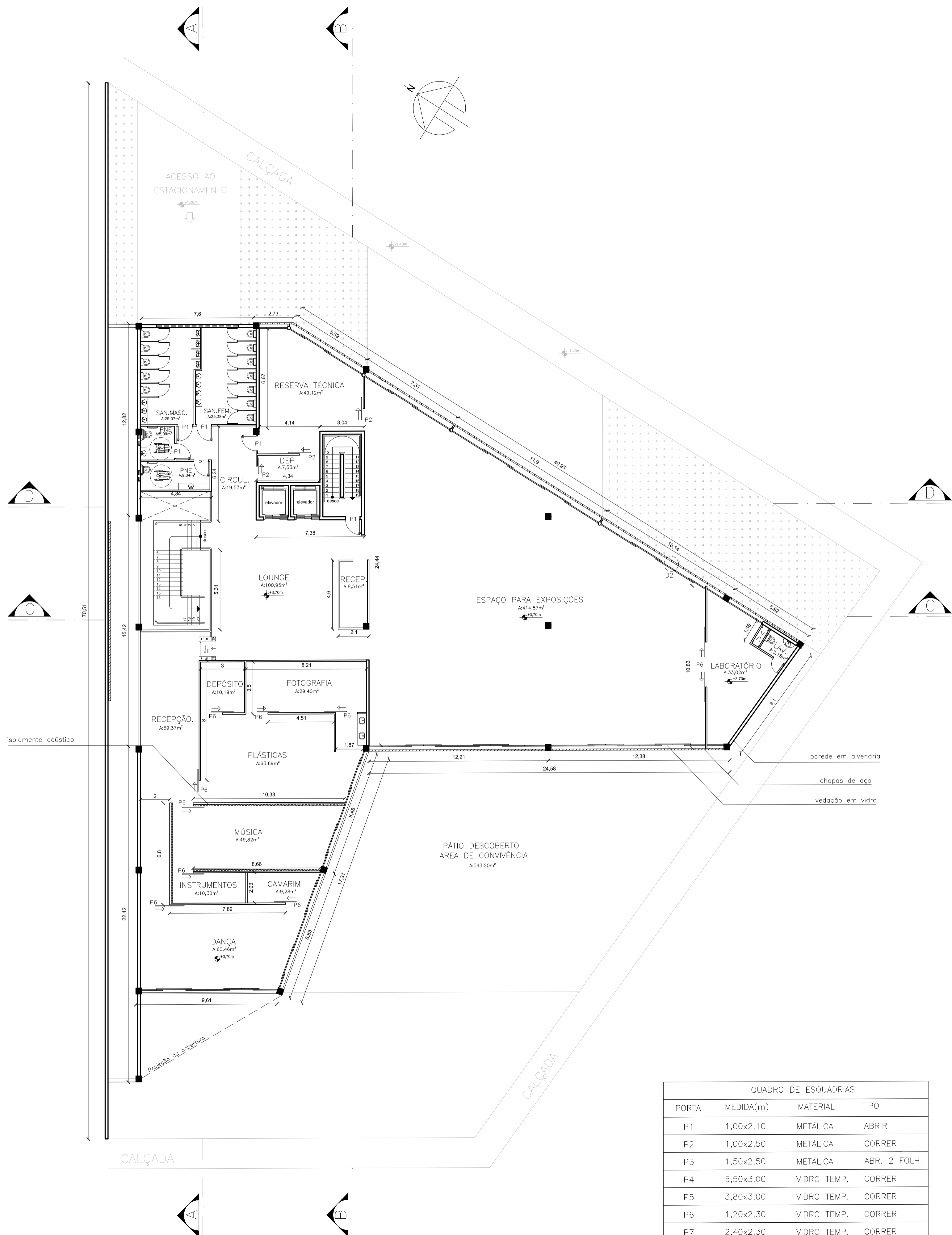
PLANTA 1º PAVIMENTO ESC: 1/125
