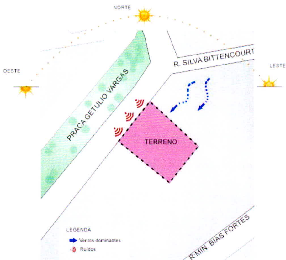
Figura 38 - Insolação, ventilação e ruídos.
