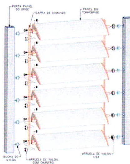
Figura 48 – Detalhe brise fachada lateral.
