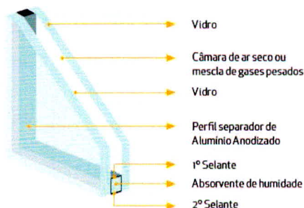
Figura 49 – Detalhe vidro duplo.
