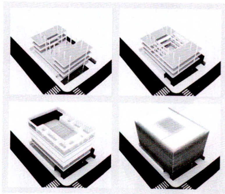
Figura 17 – Etapas construtivas, desenho autores.
