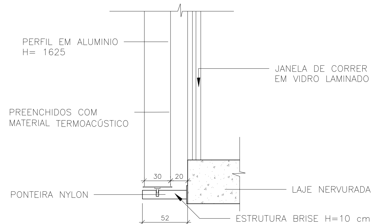
22 DETALHE BRISES VERTICAIS ESCALA 1:25
