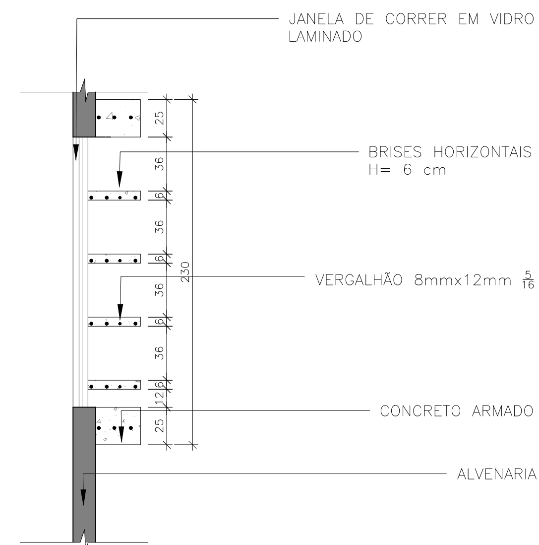
18 DETALHE BRISES HORIZONTAIS ESCALA 1:25
