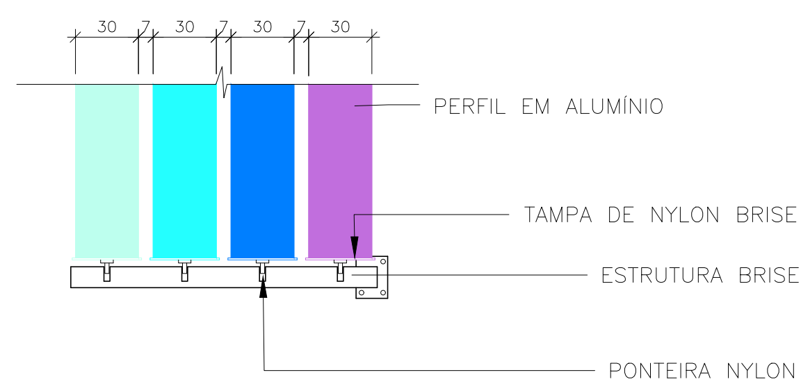
21 DETALHE BRISES VERTICAIS ESCALA 1:25
