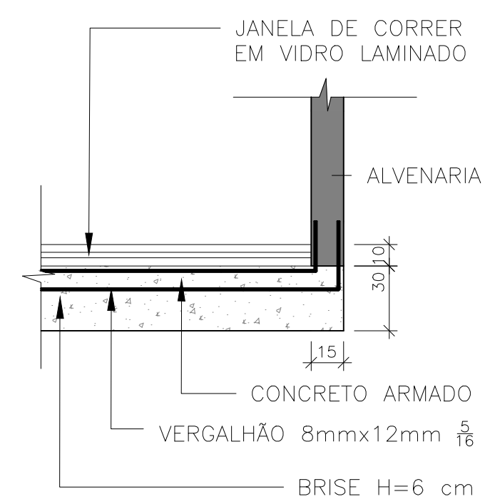
17 DETALHE BRISES HORIZONTAIS ESCALA 1:25
