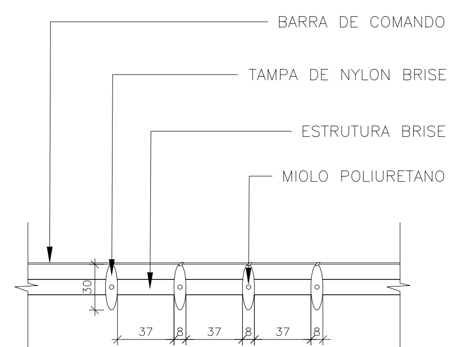
20 DETALHE BRISES VERTICAIS ESCALA 1:25
