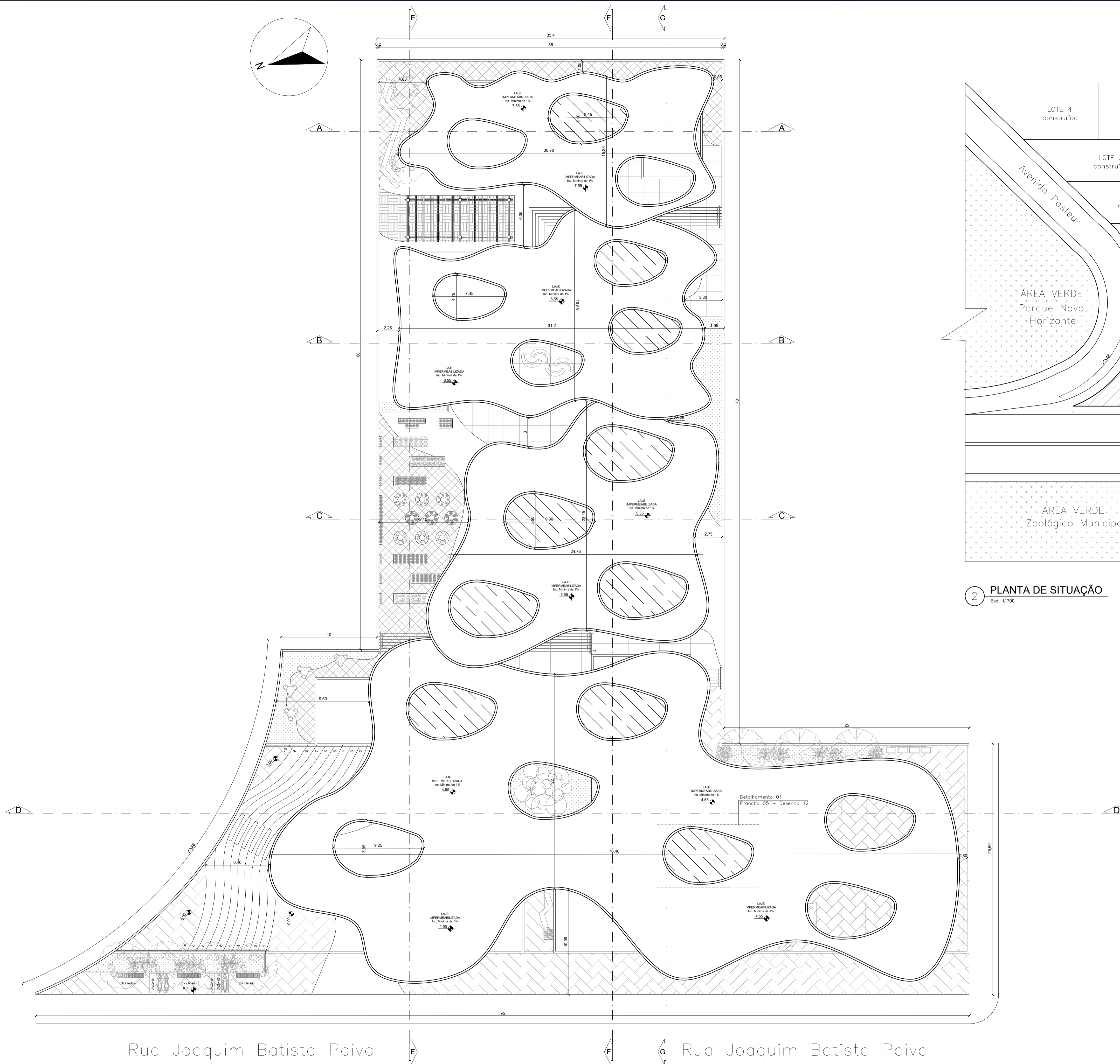
1 PLANTA DE IMPLANTAÇÃO E COBERTURA 1 Esc.: 1/200
