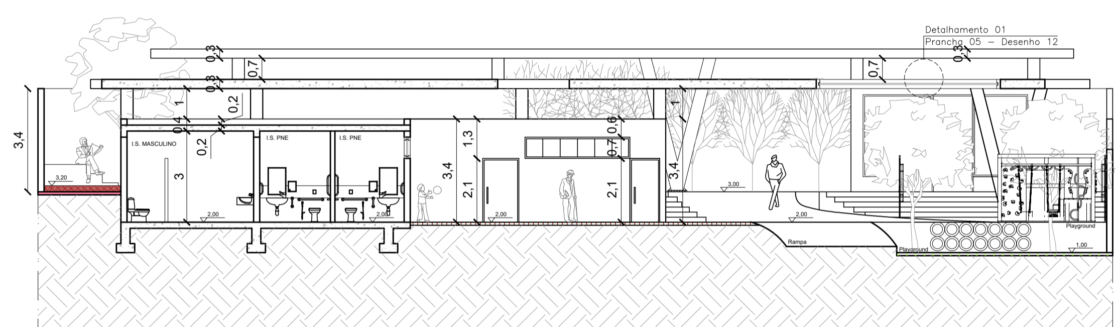
7 CORTE BB Esc: 1/125
