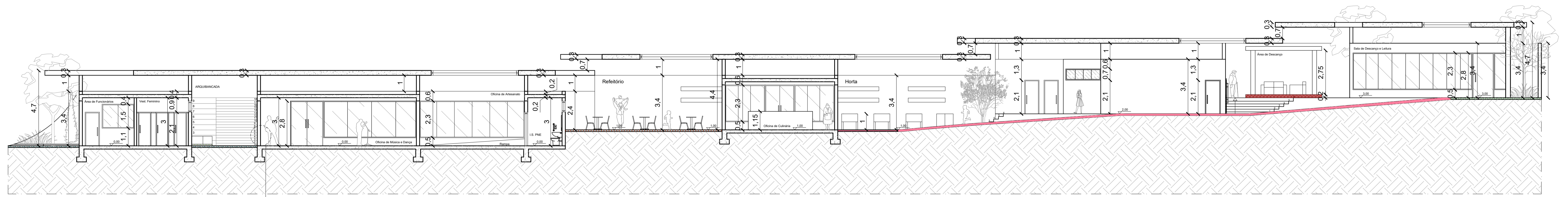
13 CORTE FF Esc.: 1/125
