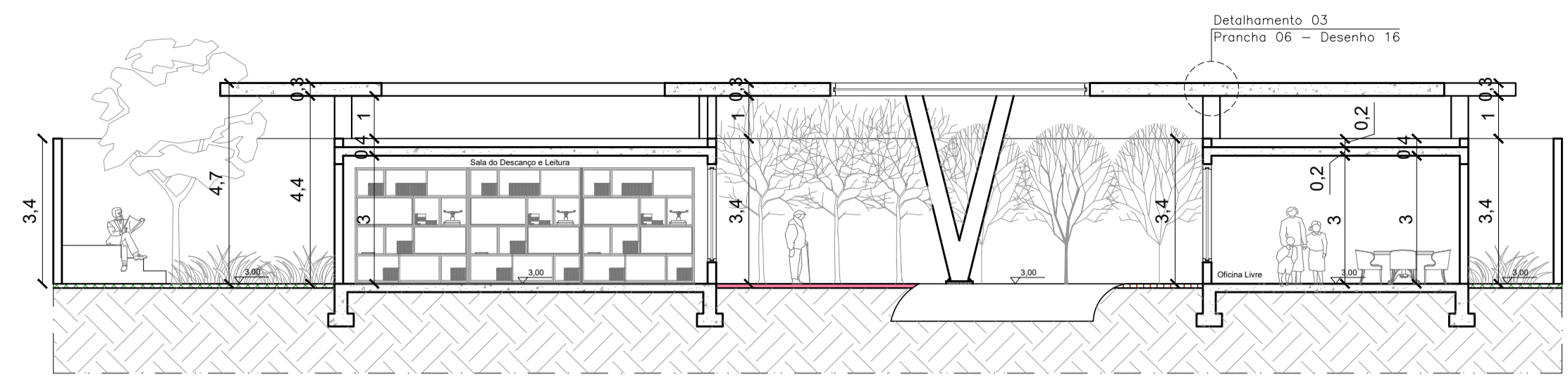
6 CORTE AA Esc: 1/125
