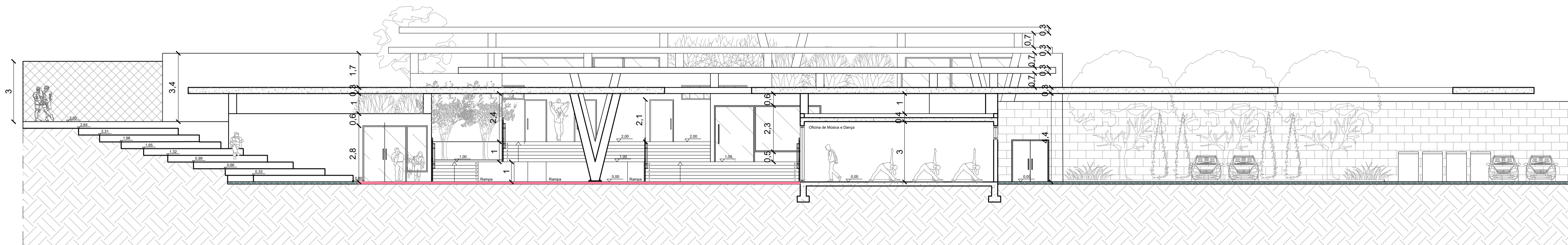
10 CORTE DD Esc.: 1/125
