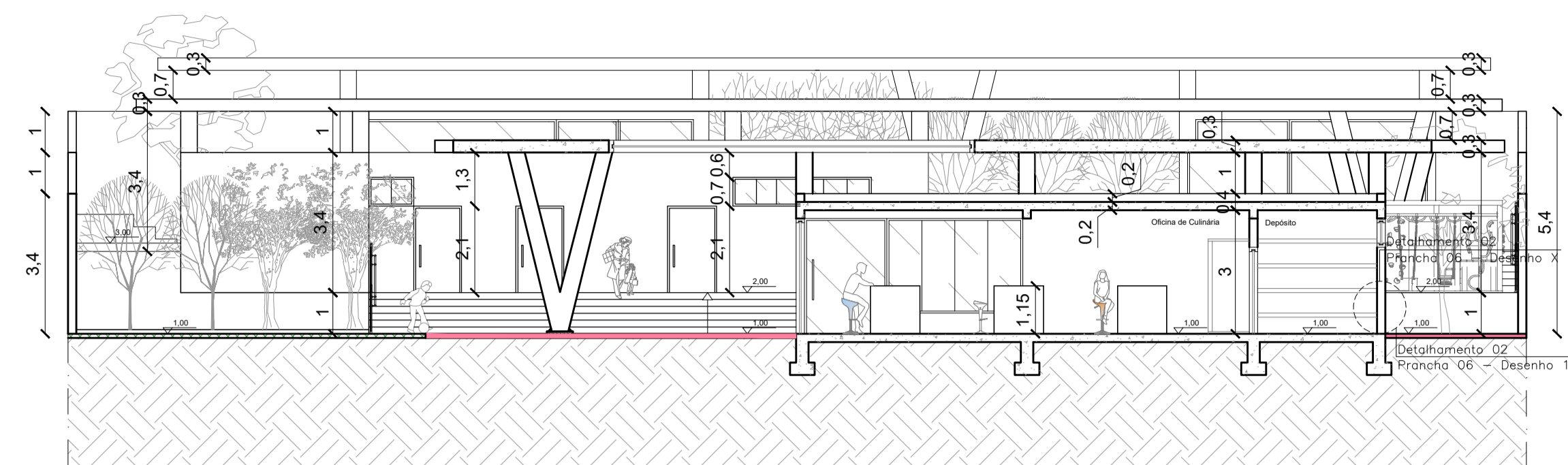
9 CORTE CC Esc.: 1/125
