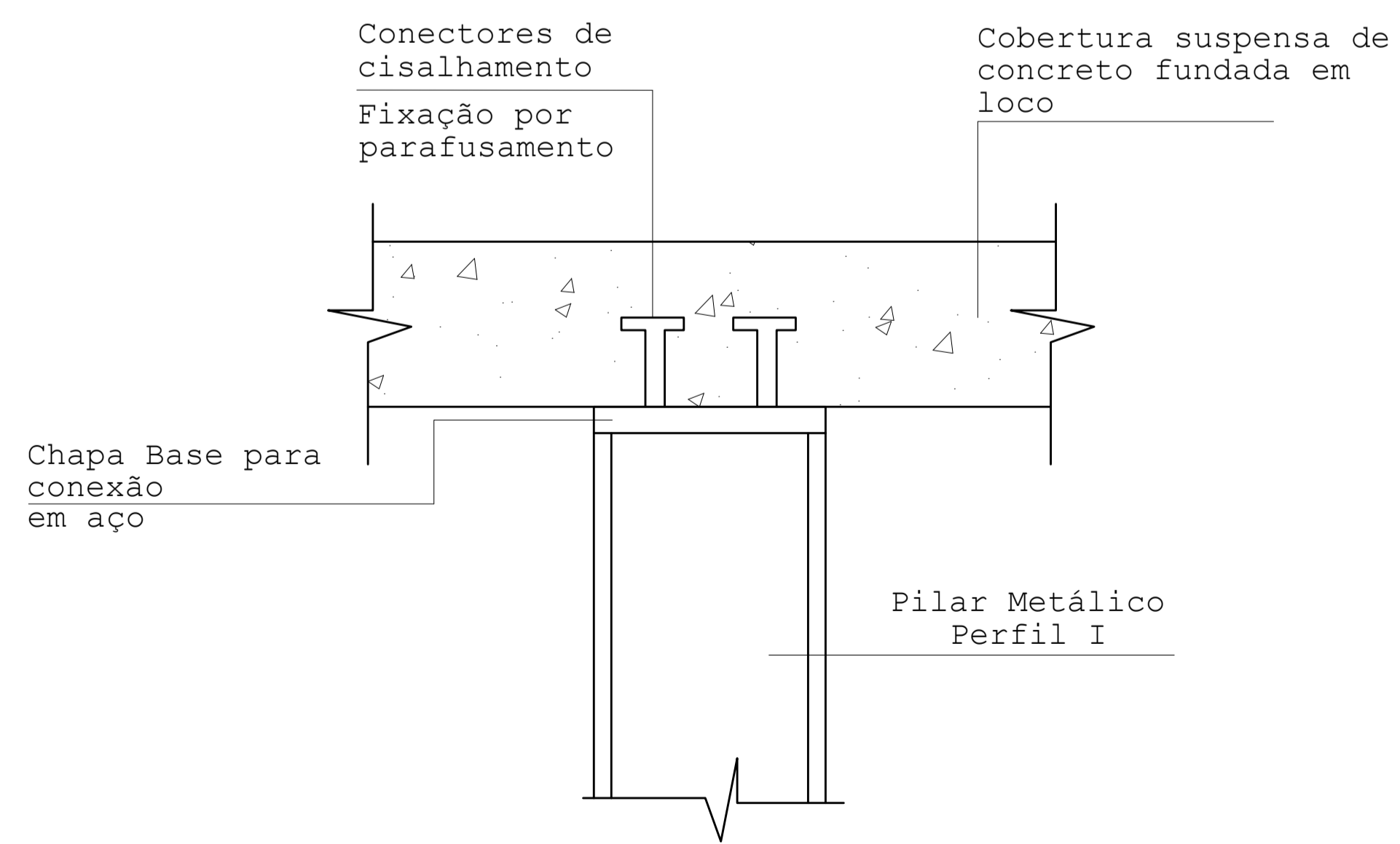
16 DETALHAMENTO 03 Esc.: 1/10
