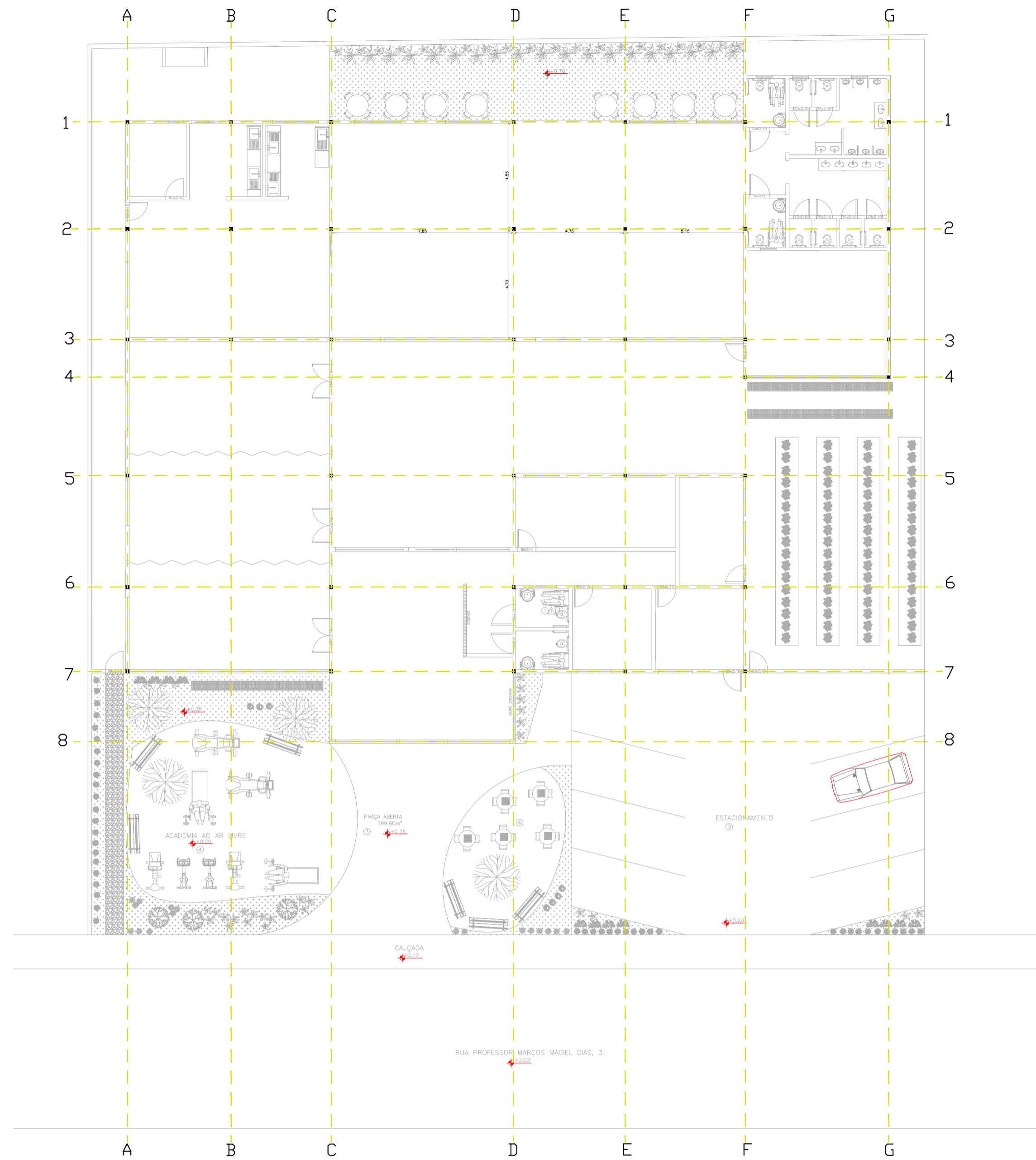
4 DIAGRAMA ESTRUTURAL ESCALA 1/150
