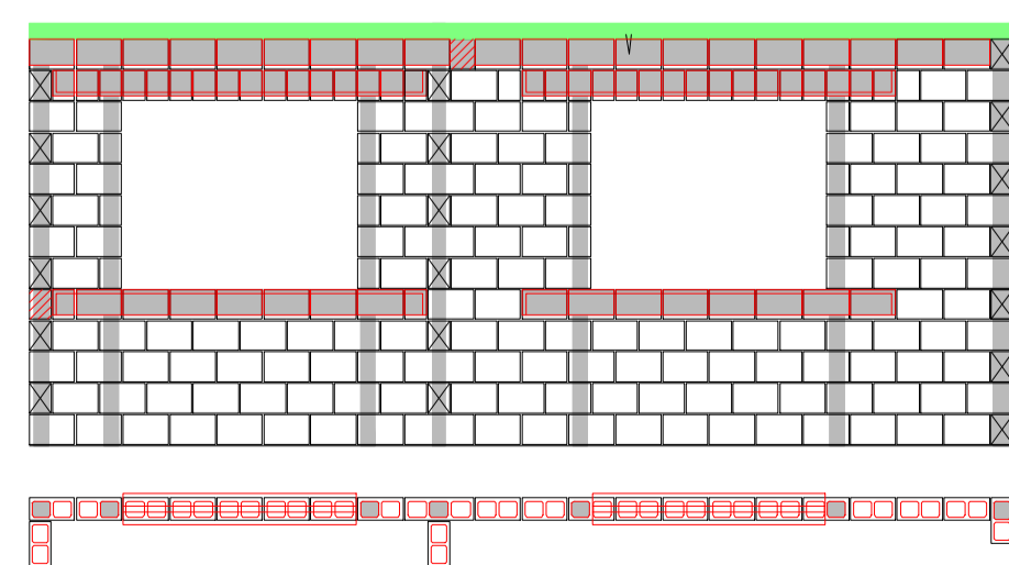
DETALHAMENTO ALVENARIA S/ ESCALA
