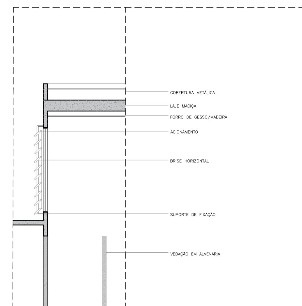
DET 02 FIXAÇÃO DO BRISE HORIZONTAL NA ESTRUTURA esc 1:20
