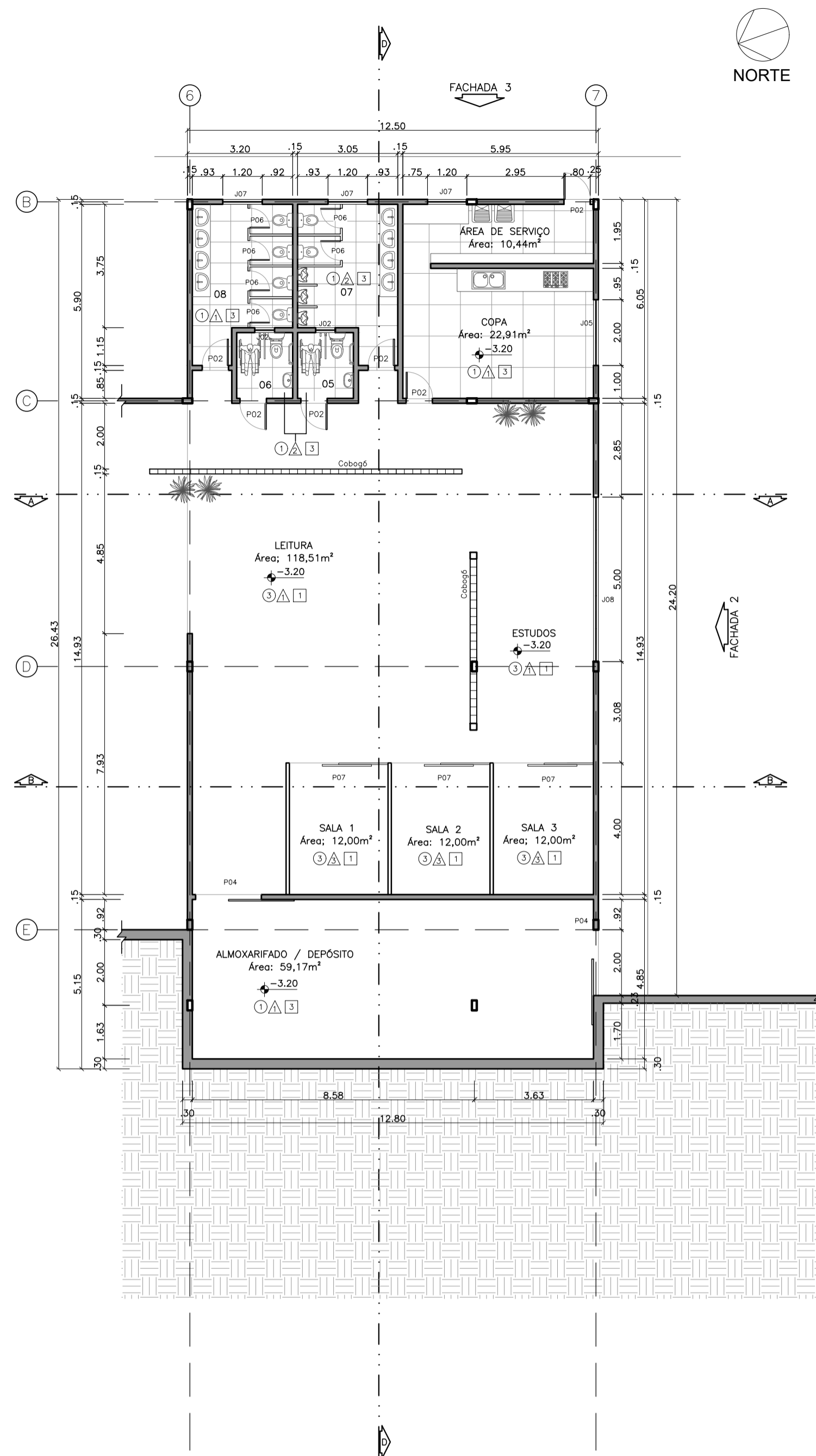
7 PLANTA PAVIMENTO SUBSOLO esc 1:125
