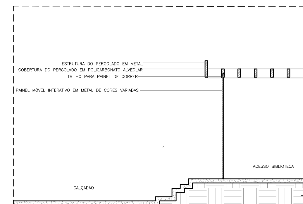
DET 01 LIGAÇÃO PAINEL PERGOLADO esc 1:20
