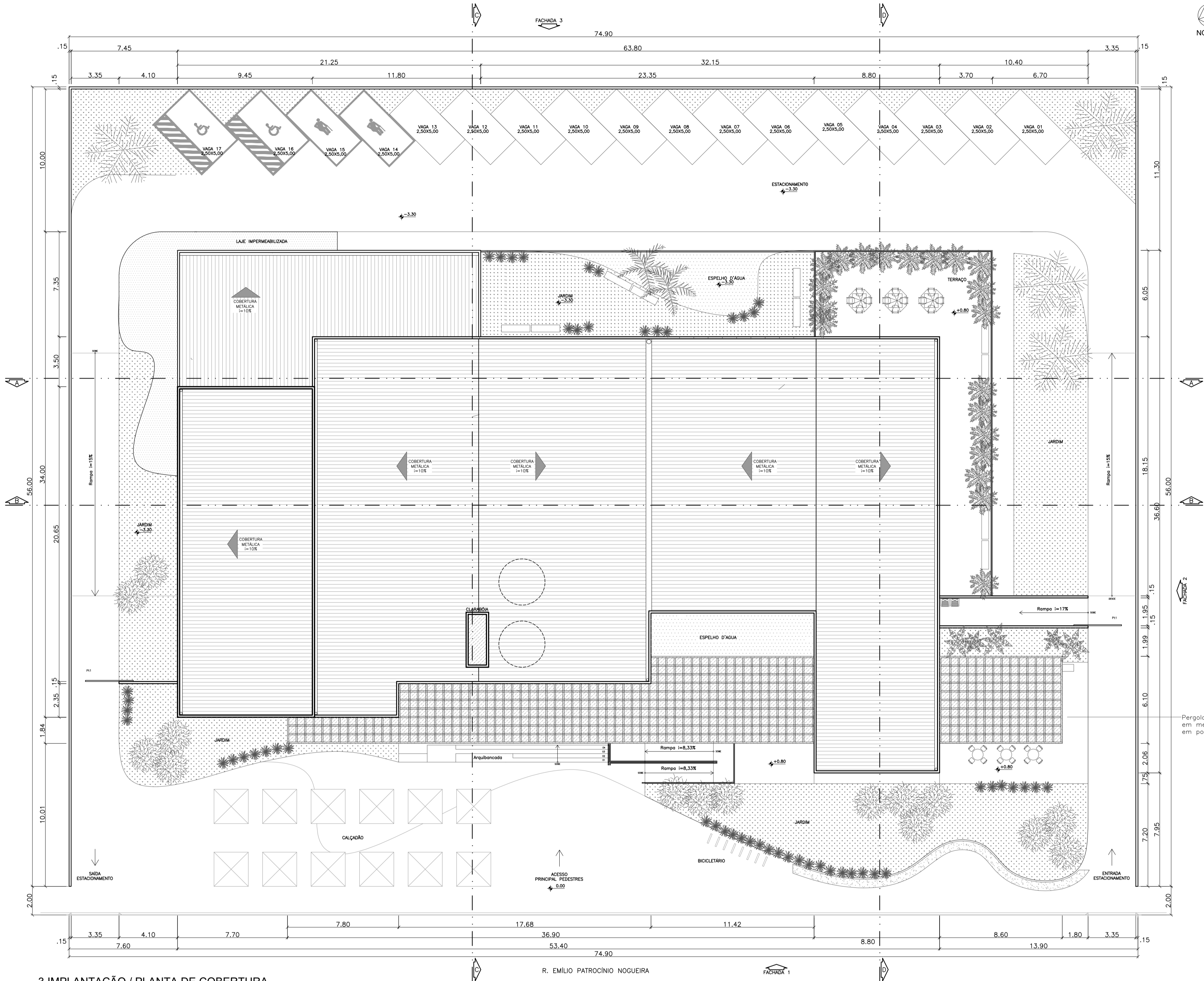
3 IMPLANTAÇÃO / PLANTA DE COBERTURA esc 1:200
