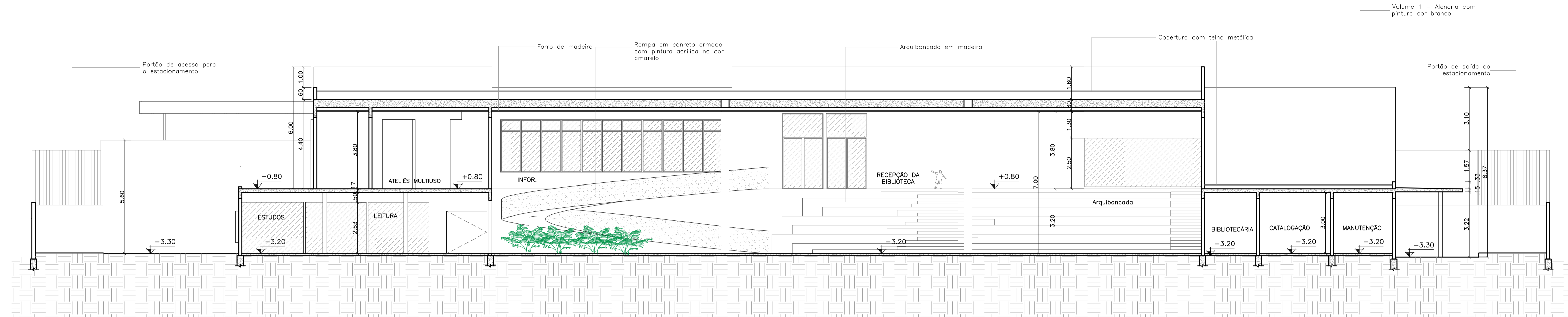
15 CORTE A esc 1:125
