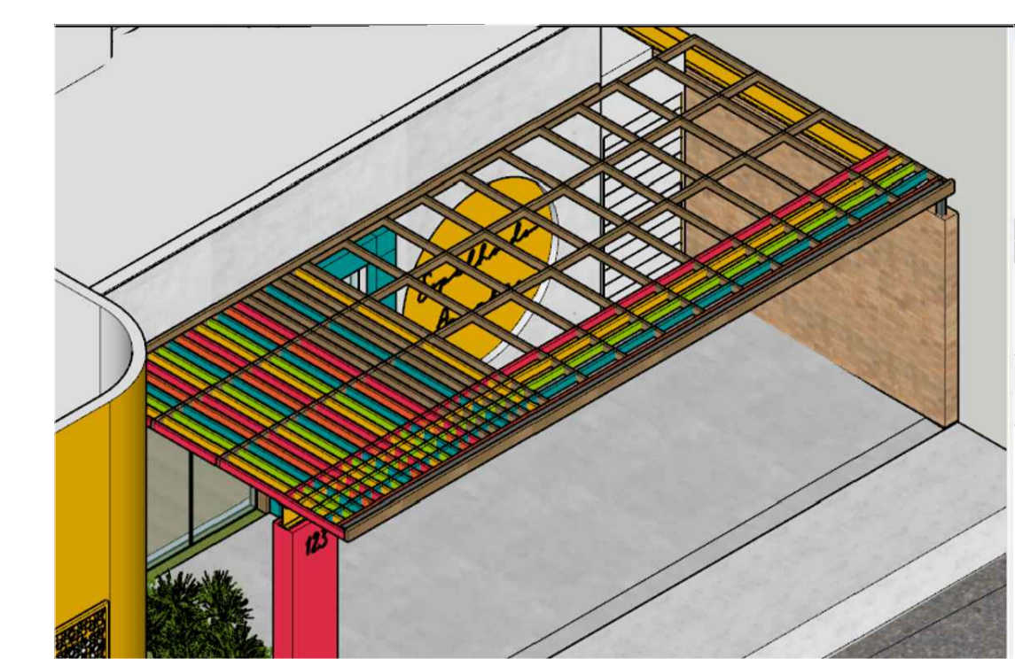
PERSPECTIVA ISOMÉTRICA COBERTURA PERGOLADO SEM POLICARBONATO PARA VISUALIZAÇÃO DAS PEÇAS DE MADEIRA (VIDE INDICAÇÃO DE CORES NO DETALHE 1B)
