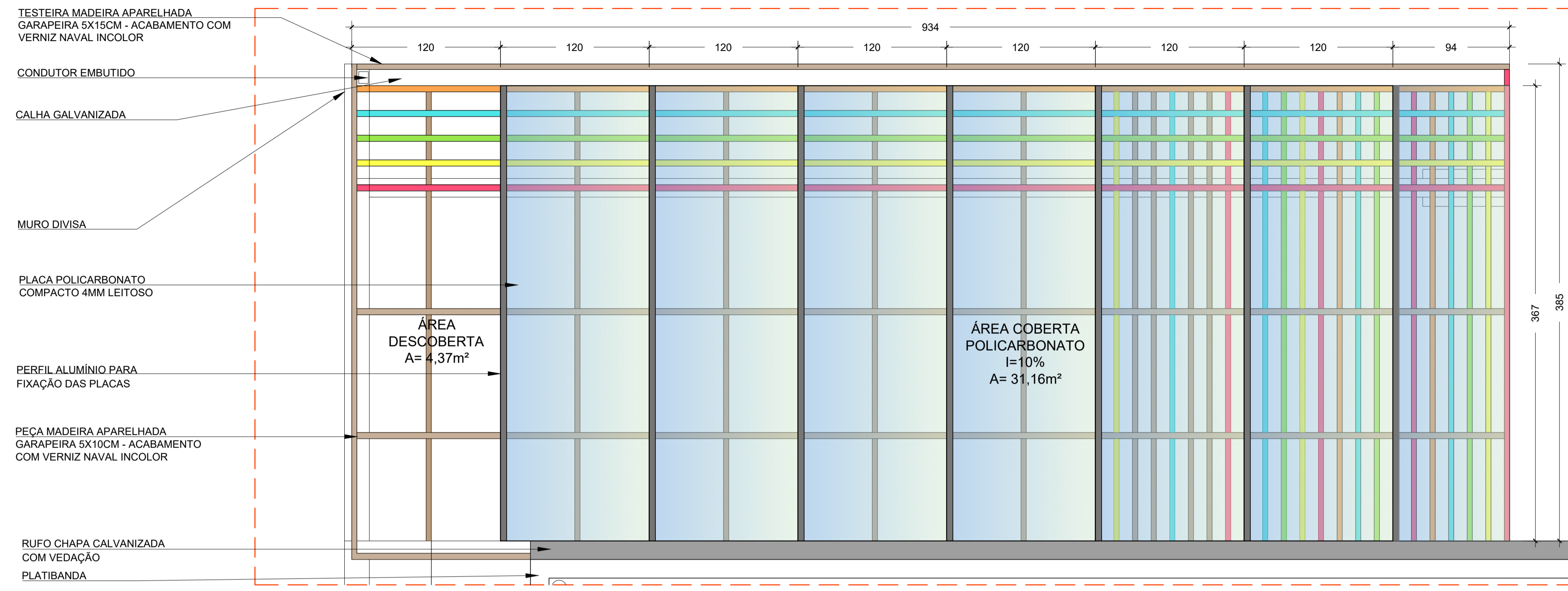
DETALHE 1A - COBERTURA POLICARBONATO + PERGOLADO ESCALA: 1/25
