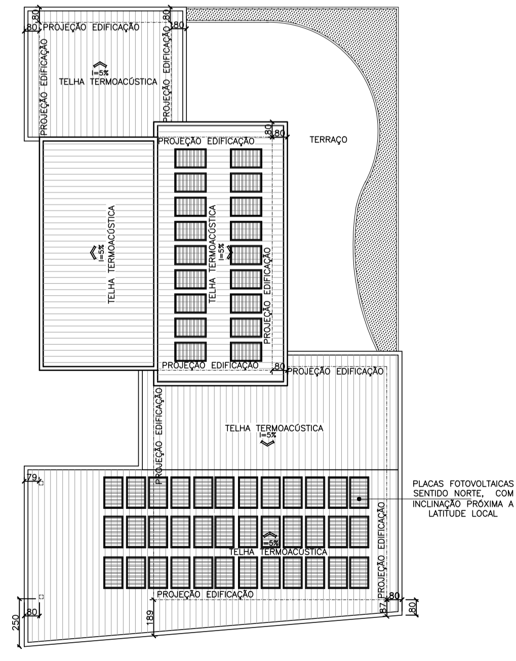
PLANTA BAIXA COBERTURA esc 1:200
