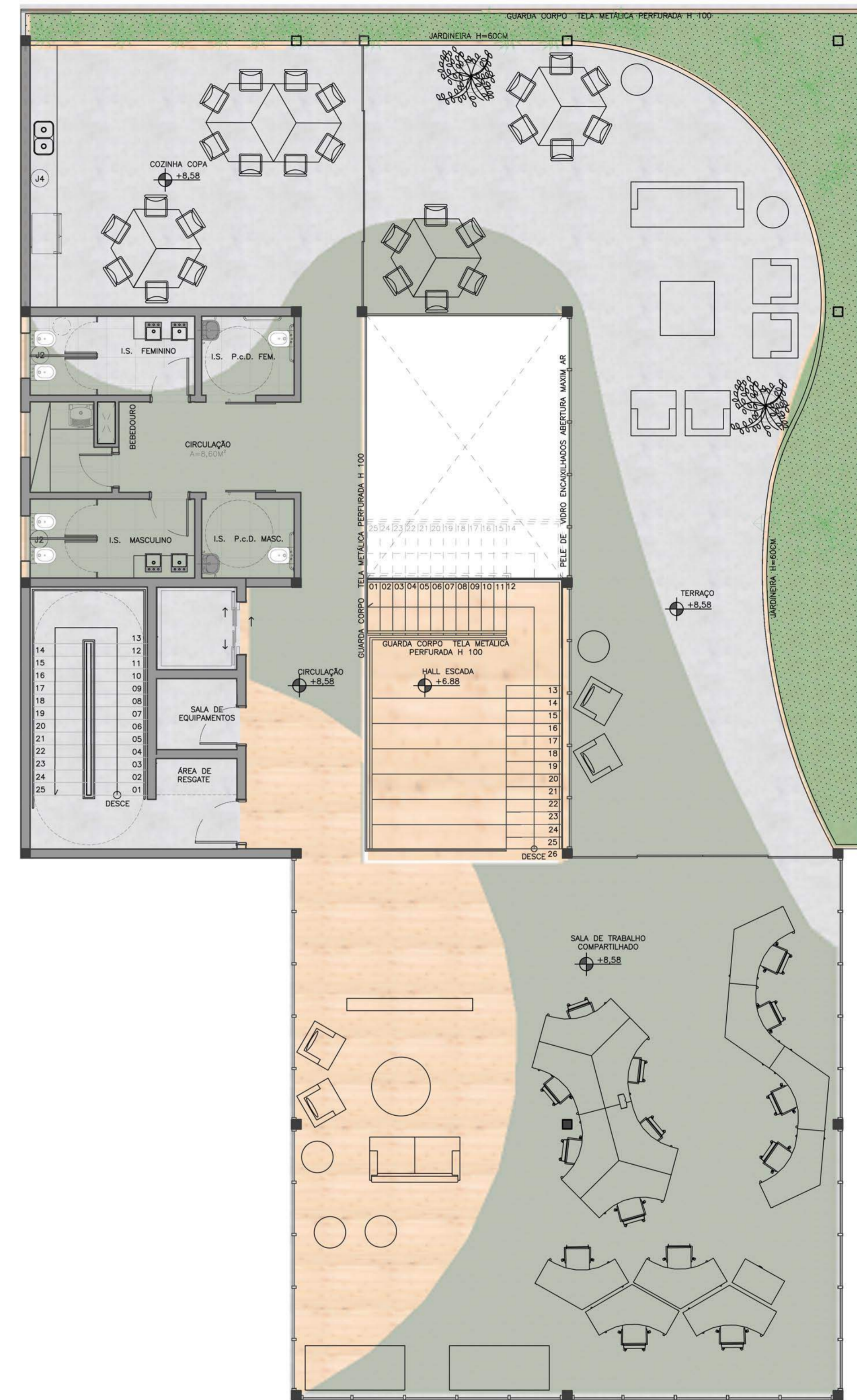
PLANTA BAIXA HUMANIZADA SEGUNDO PAVIMENTO ESC. 1:75
