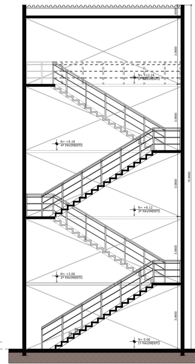
04 CORTE CD - TIROLESA ESCALA 1:100
