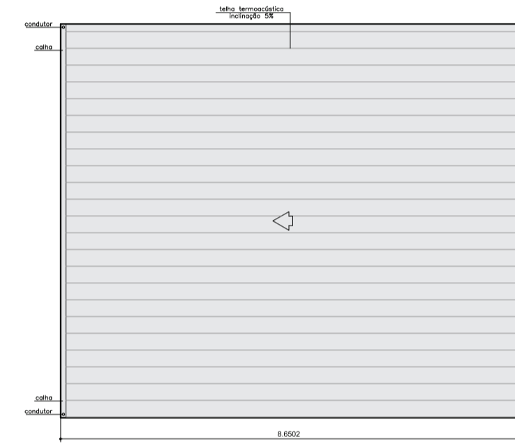
02 PLANTA COBERTURA - SANITÁRIO 2/3 ESCALA 1:100
