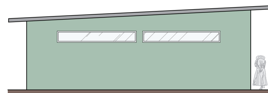
08 FACHADA POSTERIOR - SANITÁRIO 3/3 ESCALA 1:100
