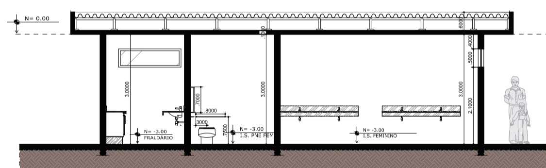
04 CORTE CD - SANITÁRIO 3/3 ESCALA 1:100
