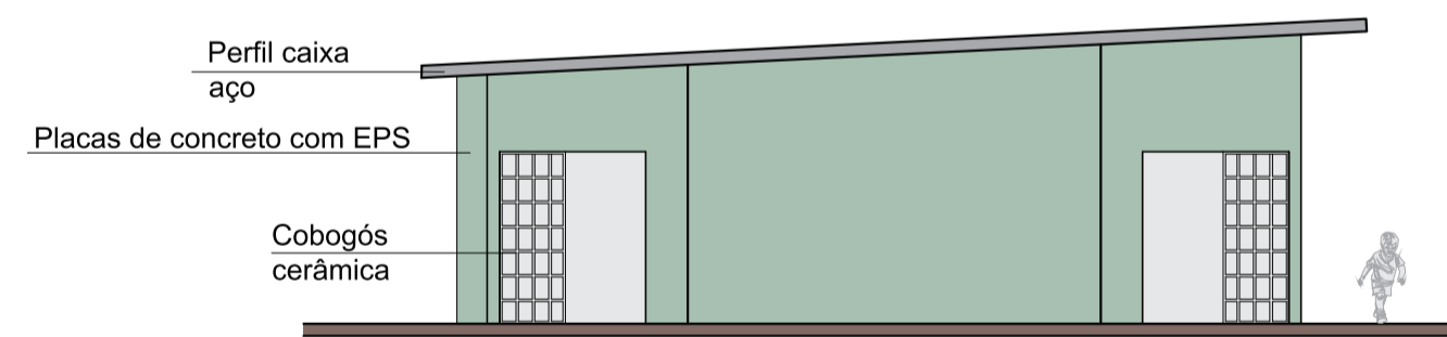
05 FACHADA FRONTAL - SANITÁRIO 3/3 ESCALA 1:100
