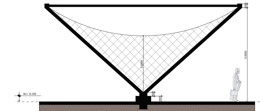
04 CORTE CD - PORTAL ESCALA 1:100
