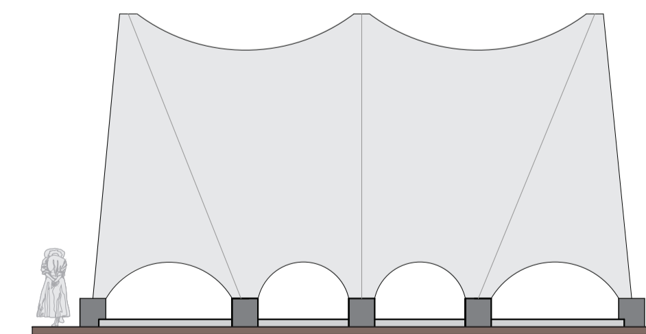
08 FACHADA POSTERIOR - PALCO DE EVENTOS ESCALA 1:100
