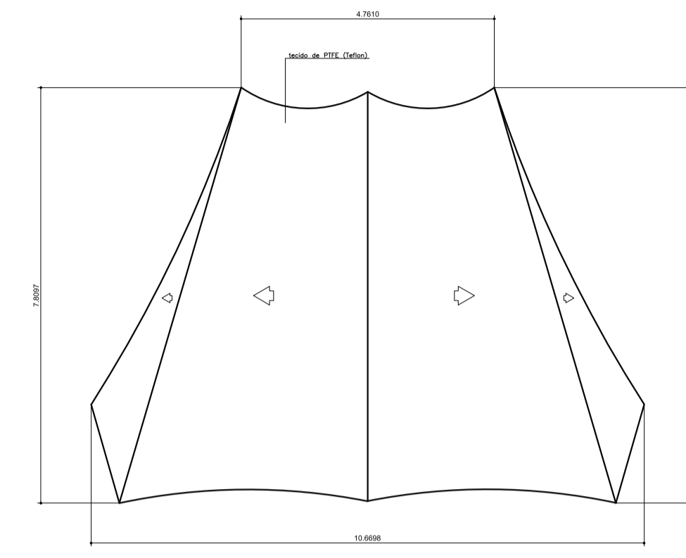
02 PLANTA COBERTURA - PALCO DE EVENTOS ESCALA 1:100
