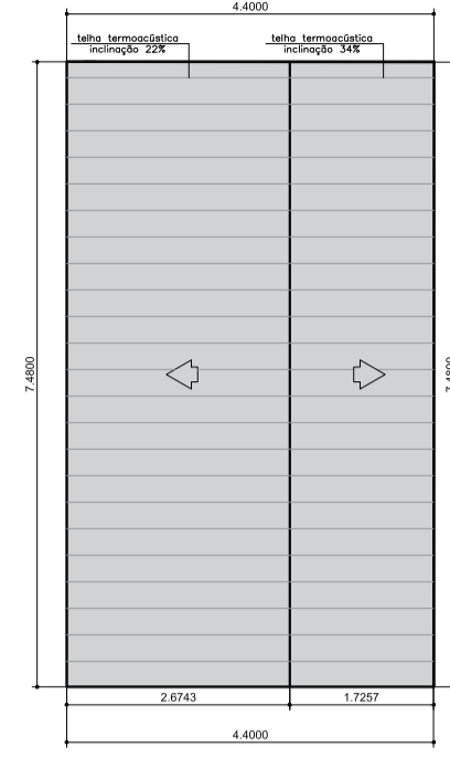
02 PLANTA COBERTURA - TIROLESA ESCALA 1:100
