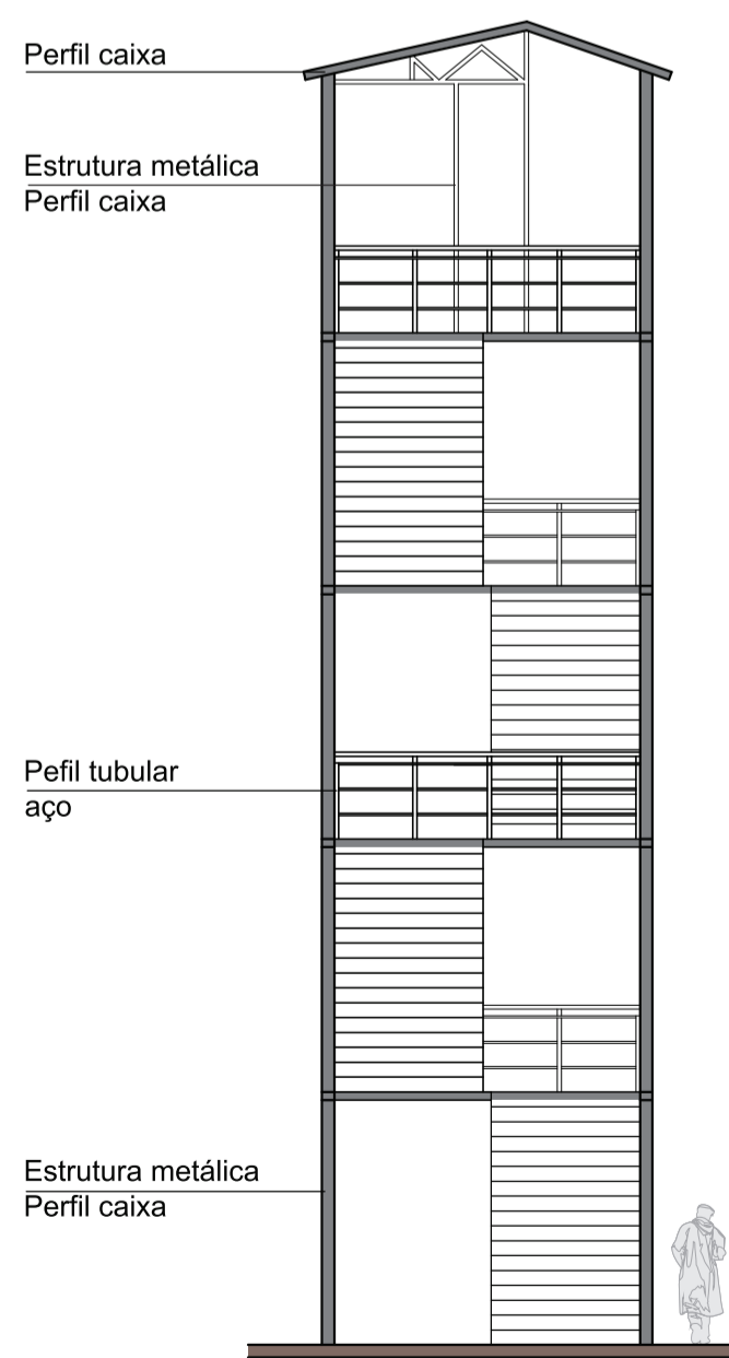
05 FACHADA FRONTAL - TIROLESA ESCALA 1:100
