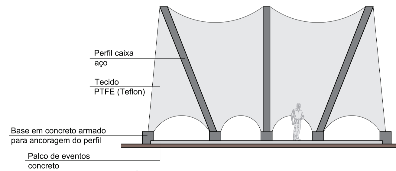
05 FACHADA FRONTAL - PALCO DE EVENTOS ESCALA 1:100
