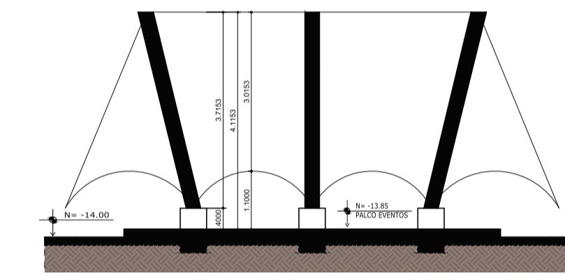
03 CORTE AB - PALCO DE EVENTOS ESCALA 1:100
