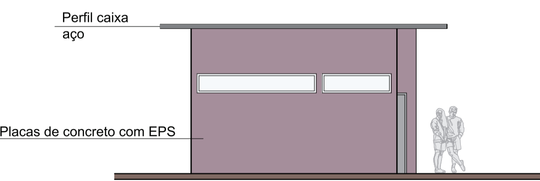
07 FACHADA DIREITA - SANITÁRIO 2/3 ESCALA 1:100
