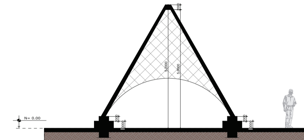
03 CORTE AB - PORTAL ESCALA 1:100
