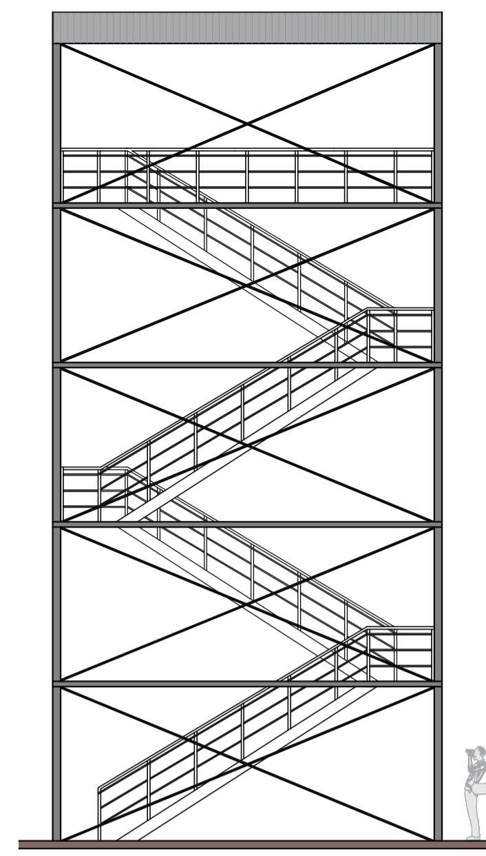
07 FACHADA DIREITA - TIROLESA ESCALA 1:100
