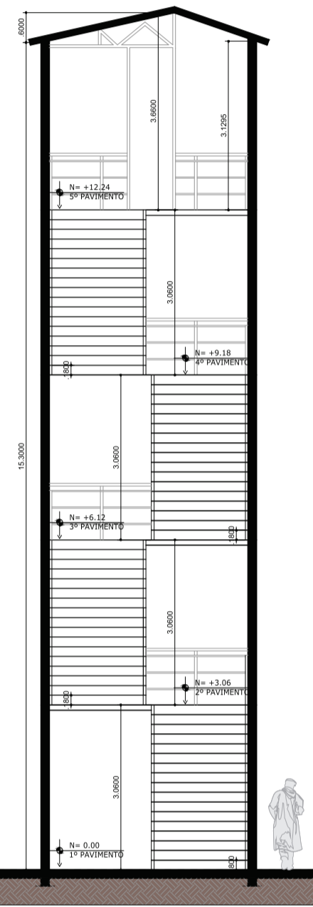
03 CORTE AB - TIROLESA ESCALA 1:100
