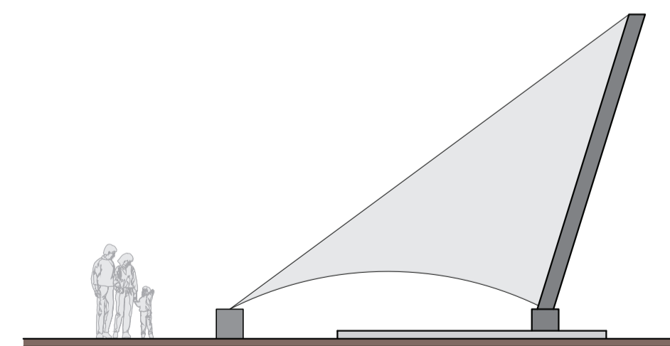
07 FACHADA DIREITA - PALCO DE EVENTOS ESCALA 1:100
