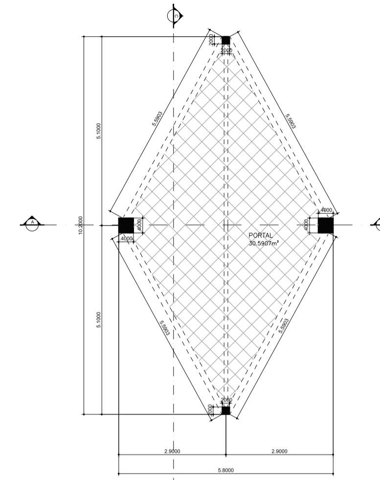
01 PLANTA - PORTAL ESCALA 1:100
