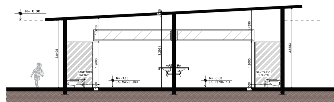
03 CORTE AB - SANITÁRIO 3/3 ESCALA 1:100
