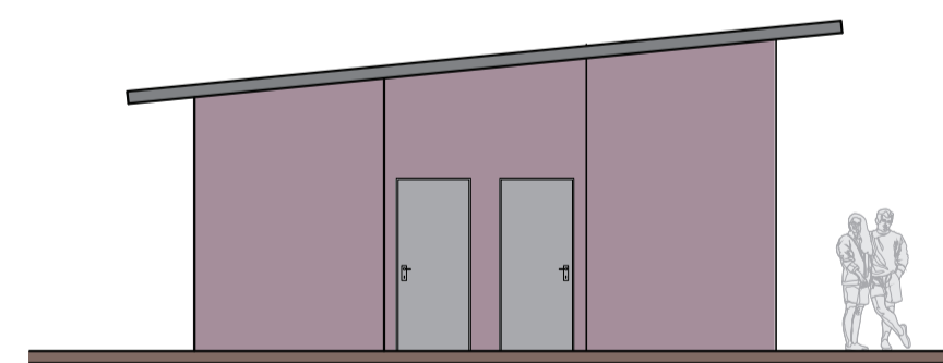
05 FACHADA FRONTAL - SANITÁRIO 2/3 ESCALA 1:100
