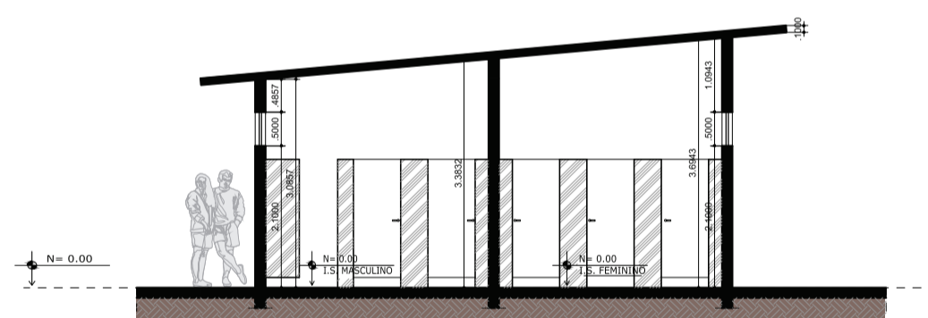
03 CORTE AB - SANITÁRIO 2/3 ESCALA 1:100
