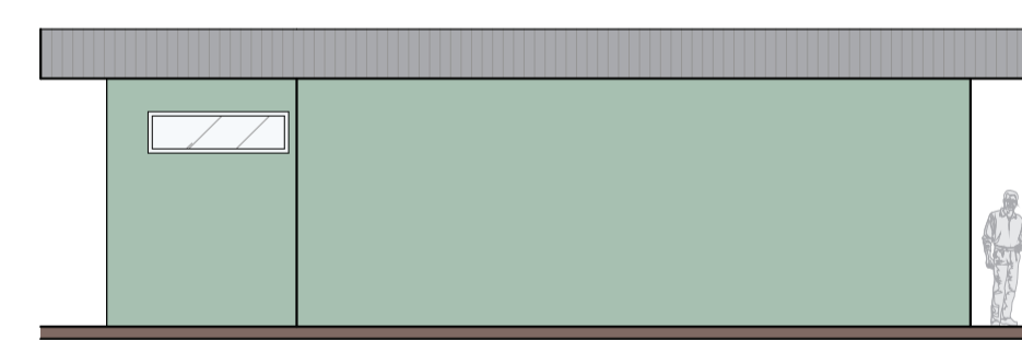
06 FACHADA ESQUERDA - SANITÁRIO 3/3 ESCALA 1:100
