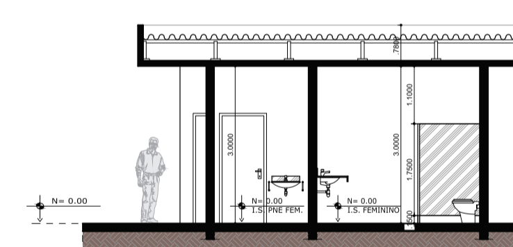
04 CORTE CD - SANITÁRIO 2/3 ESCALA 1:100
