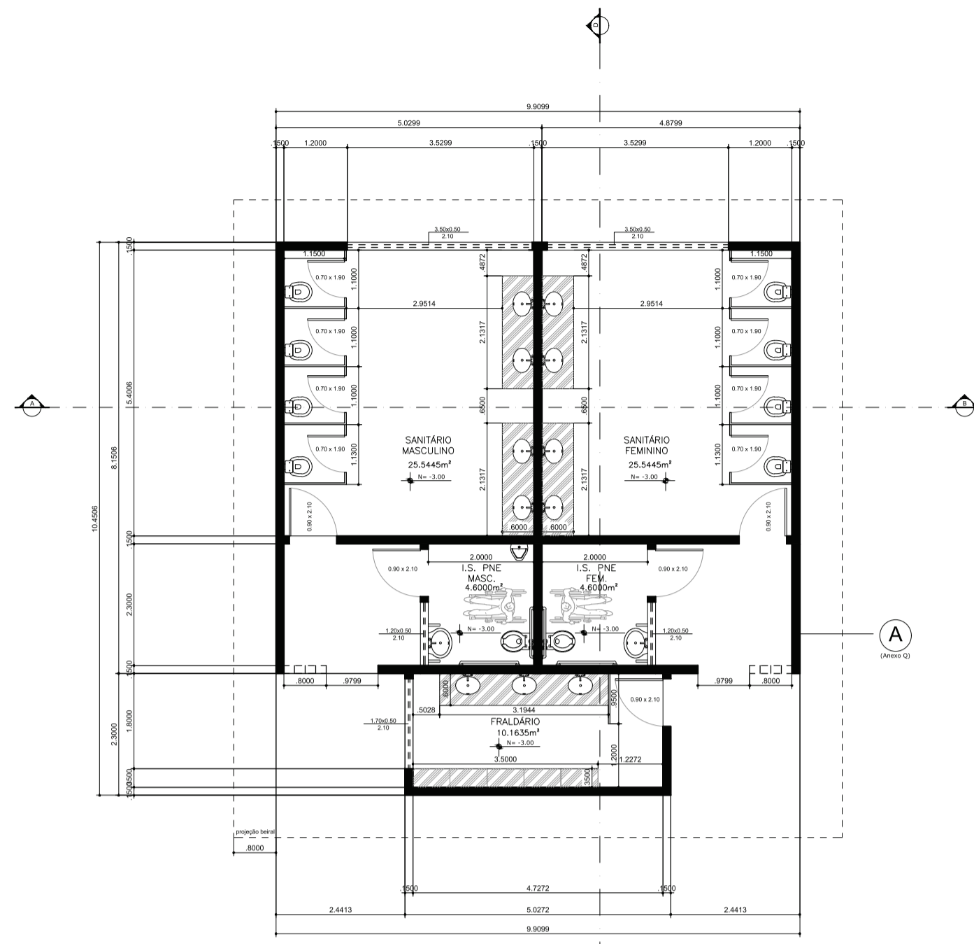
01 PLANTA - SANITÁRIO 3/3 ESCALA 1:100
