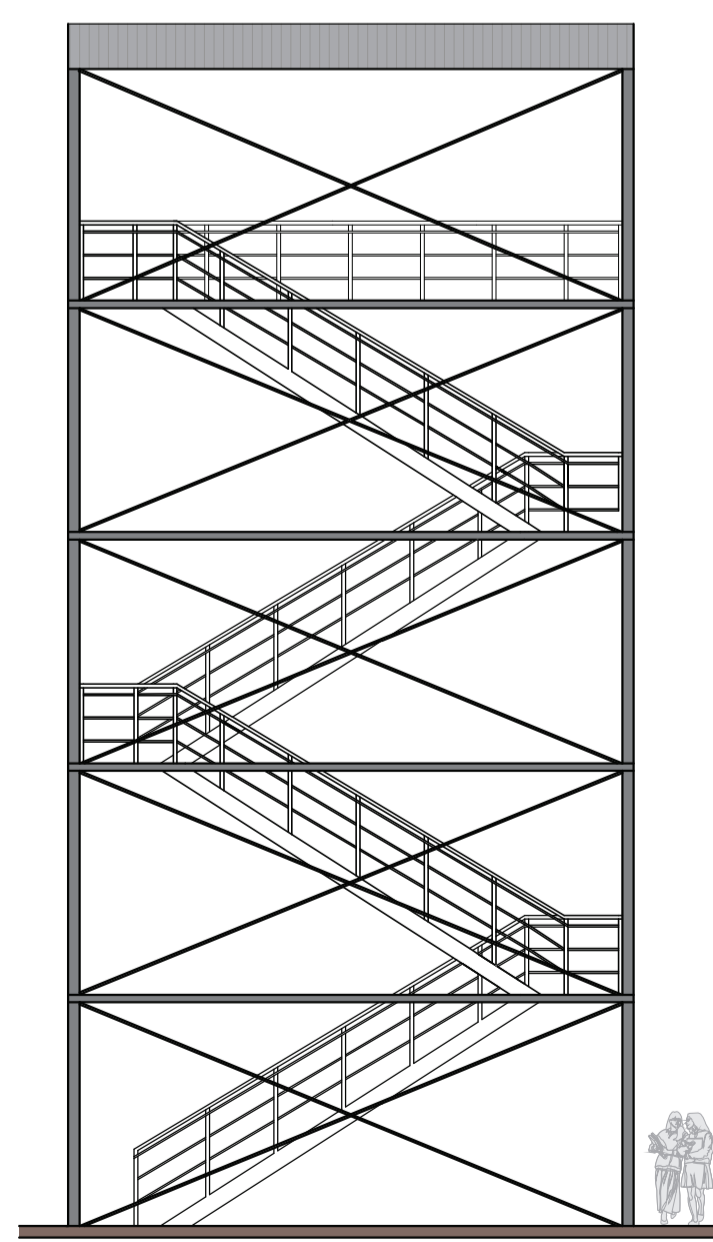
06 FACHADA ESQUERDA - TIROLESA ESCALA 1:100
