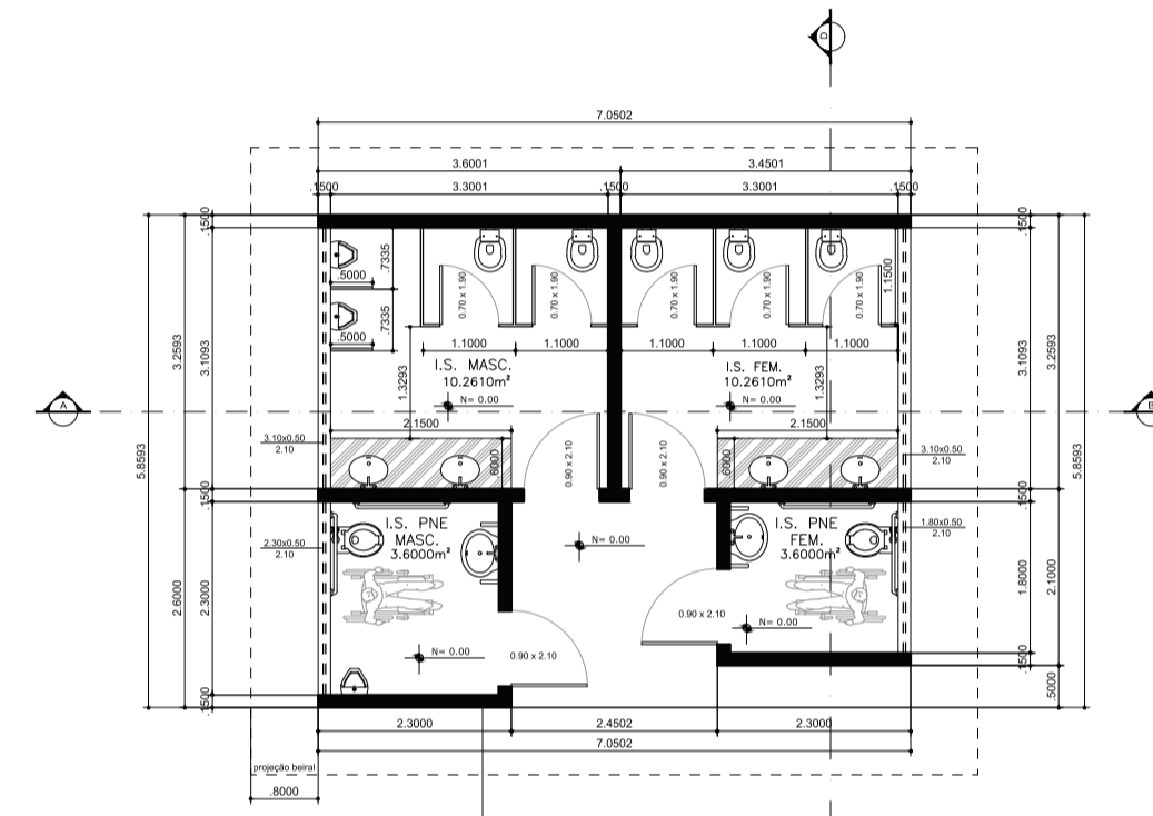
01 PLANTA - SANITÁRIO 2/3 ESCALA 1:100
