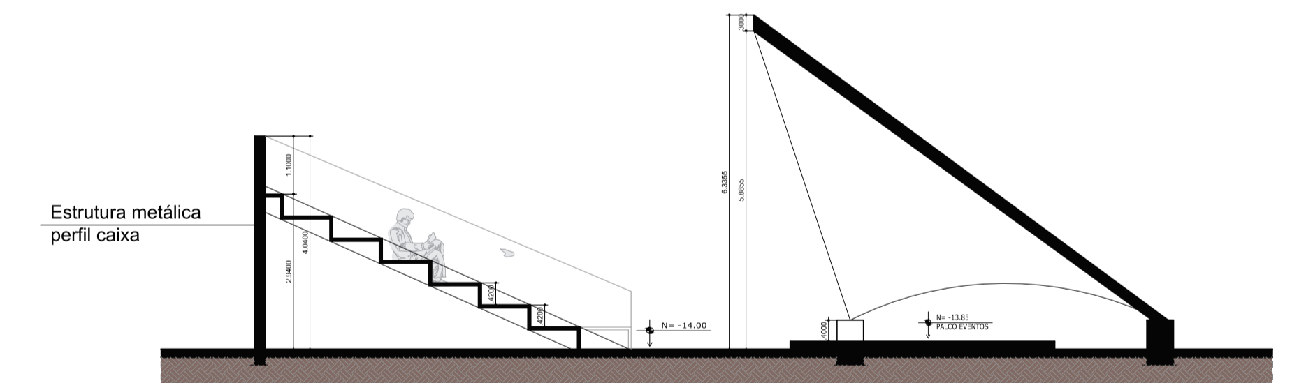
04 CORTE CD - PALCO DE EVENTOS ESCALA 1:100
