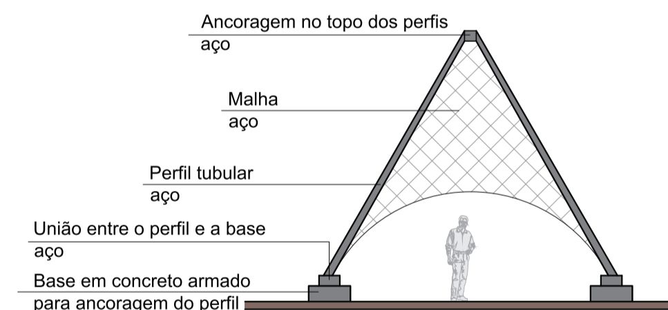
05 FACHADA FRONTAL - PORTAL ESCALA 1:100
