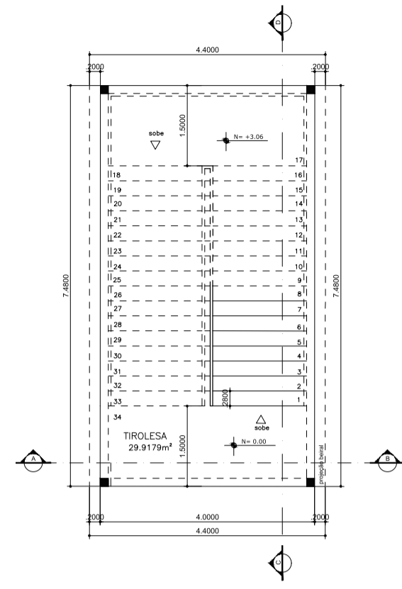
01 PLANTA - TIROLESA ESCALA 1:100
