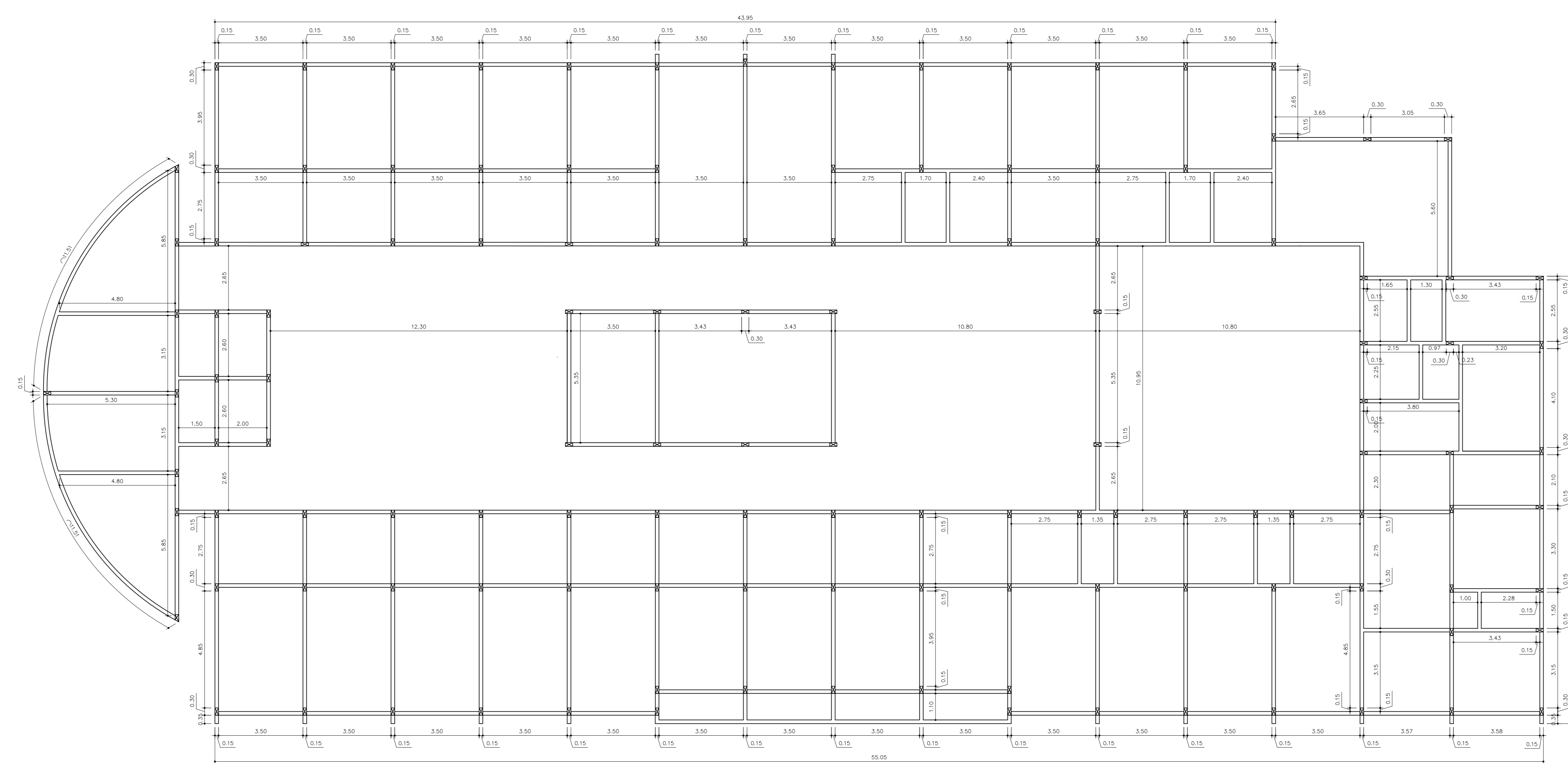
PLANTA DE FORMA PAV. SUPERIOR Escala 1/100
