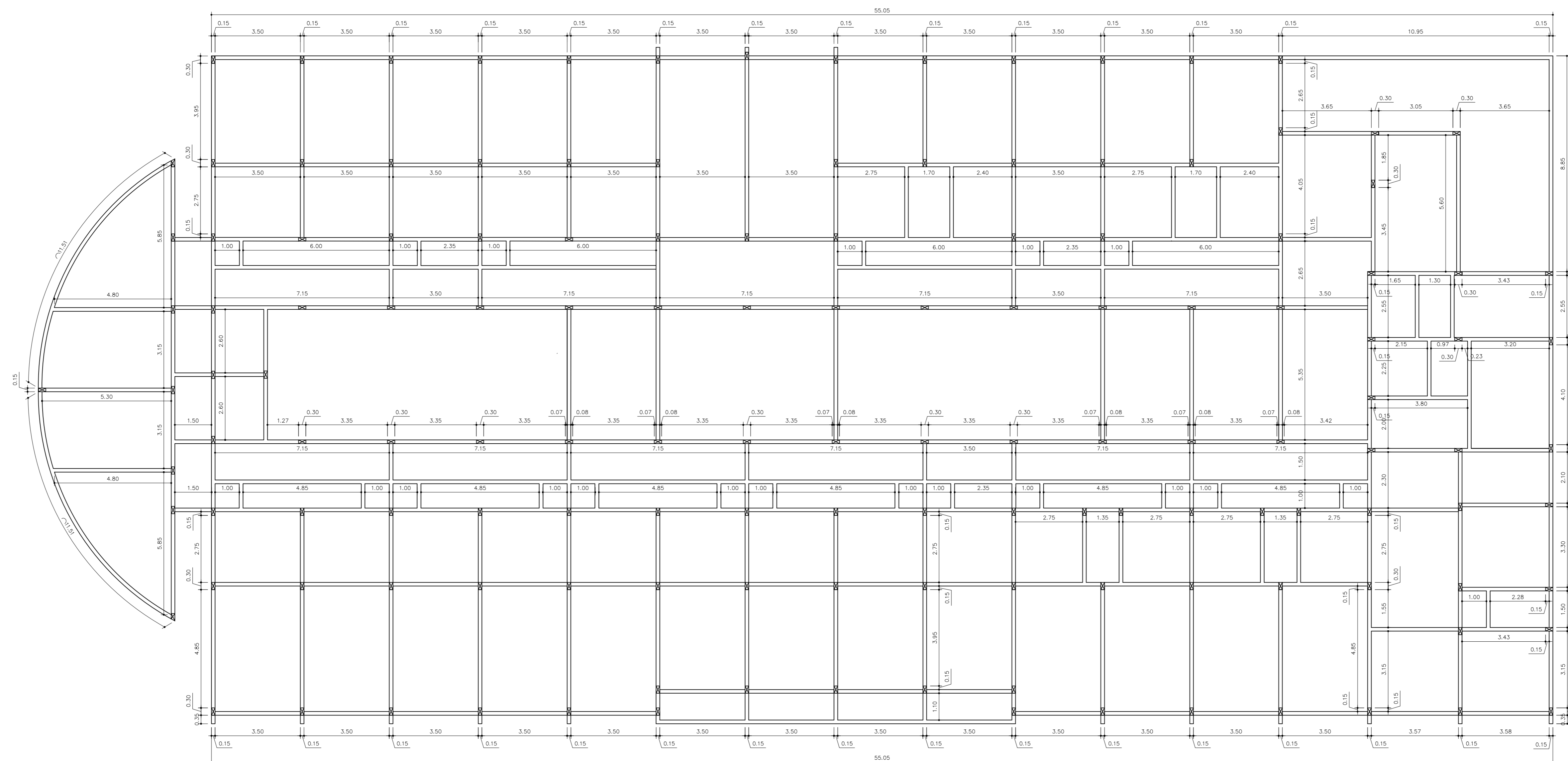
PLANTA DE FORMA PAV. TÉRREO Escala 1/100
