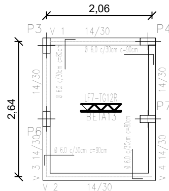
ARMAÇÃO LAJE RESERVATÓRIO (NÍVEL 750) ESC 1:75
