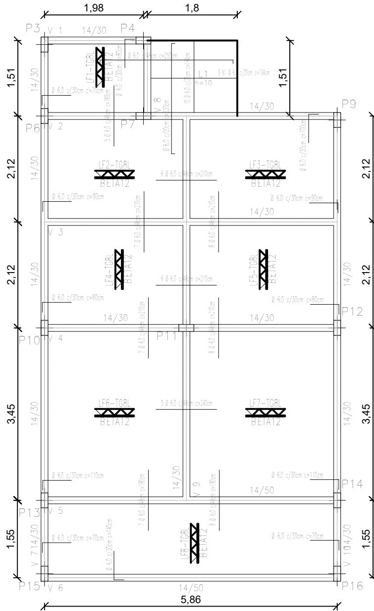
ARMAÇÃO LAJES FORRO (NÍVEL 600) ESC 1:75
