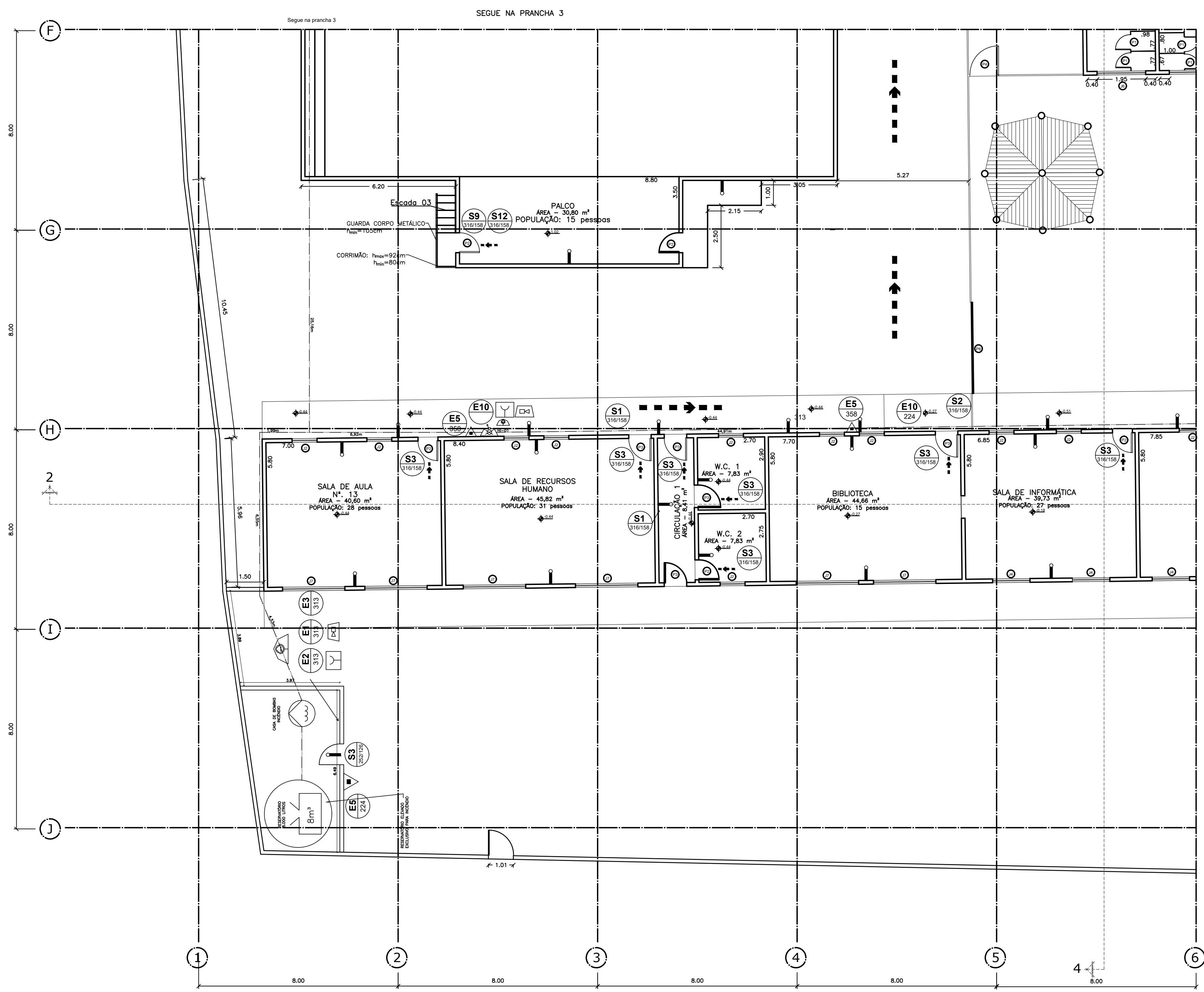
10 PLANTA BAIXA (parte III) ESCALA 1:100
