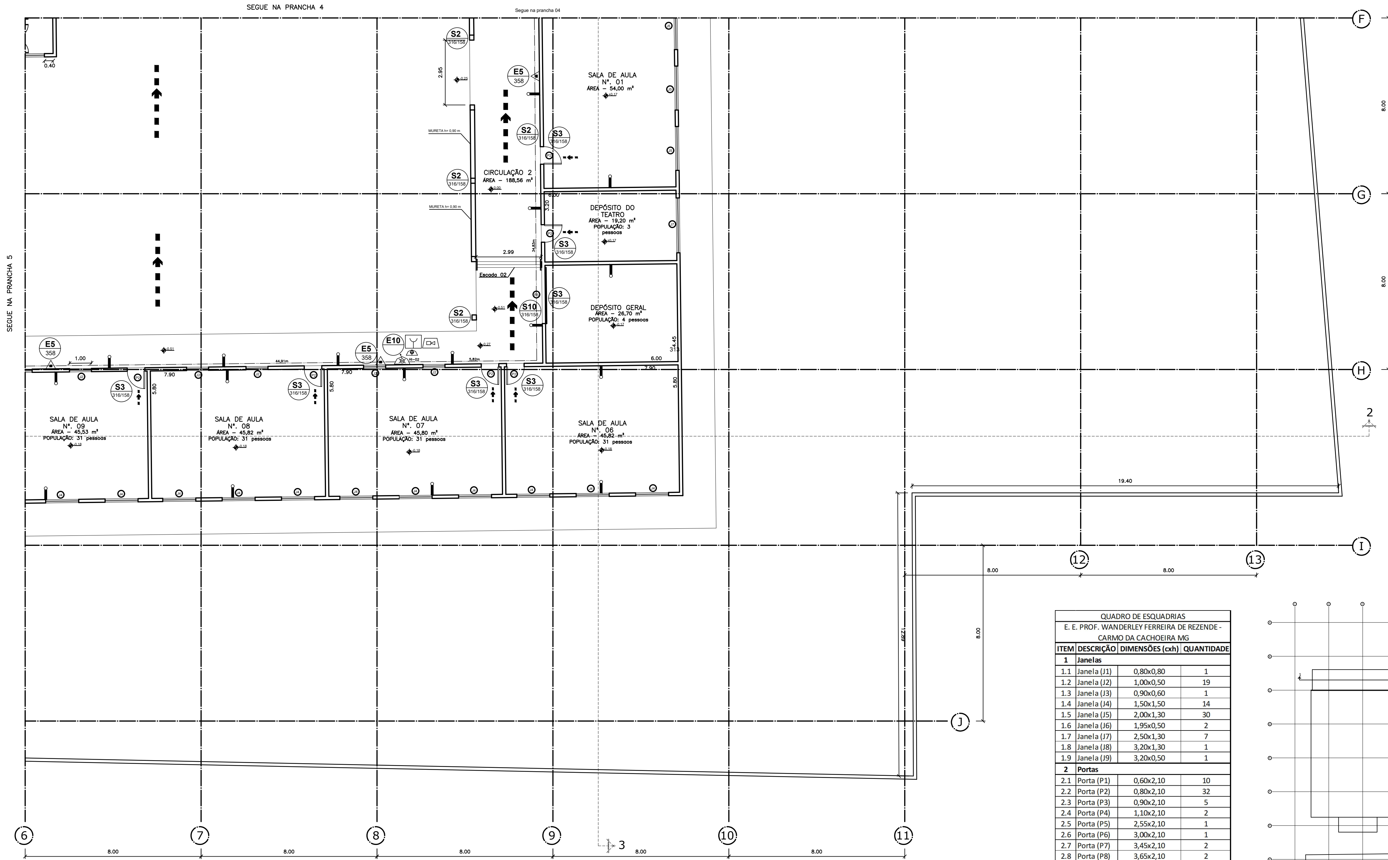
11 PLANTA BAIXA (parte IV) ESCALA 1:100
