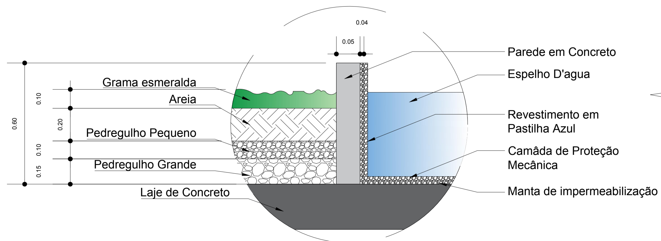
DET. JARDIM E ESPELHO D'AGUA - TERRAÇO ESCALA: SEM ESCALA
