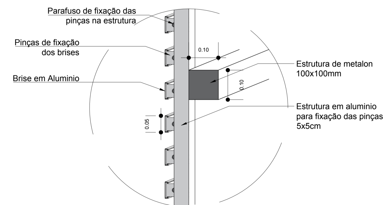
DETALHAMENTO BRISE ESCALA: SEM ESCALA
