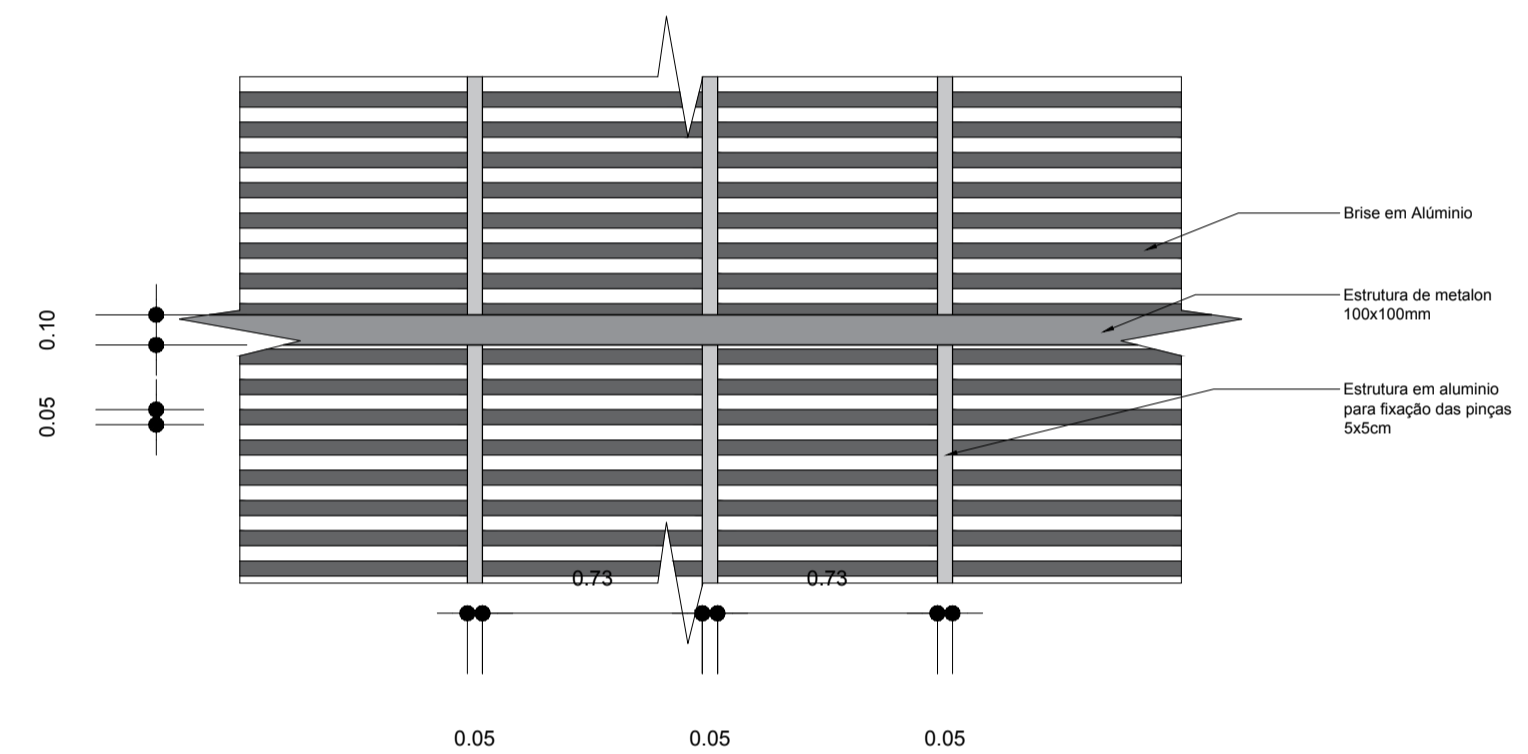
25 DET. BRISE VISTA FUNDO ESCALA: 1/25
