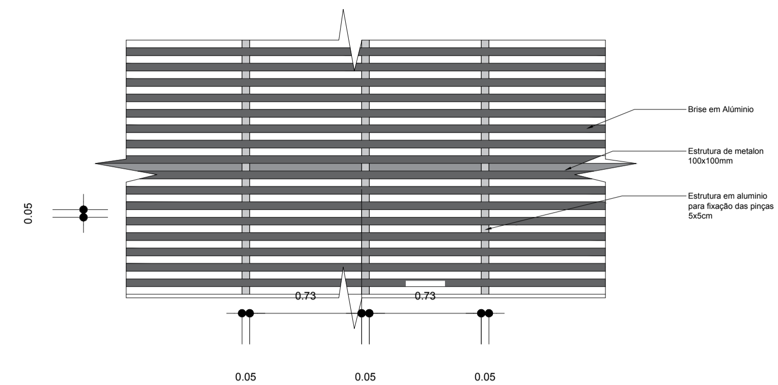
24 DET. BRISE VISTA FRONTAL ESCALA: 1/25
