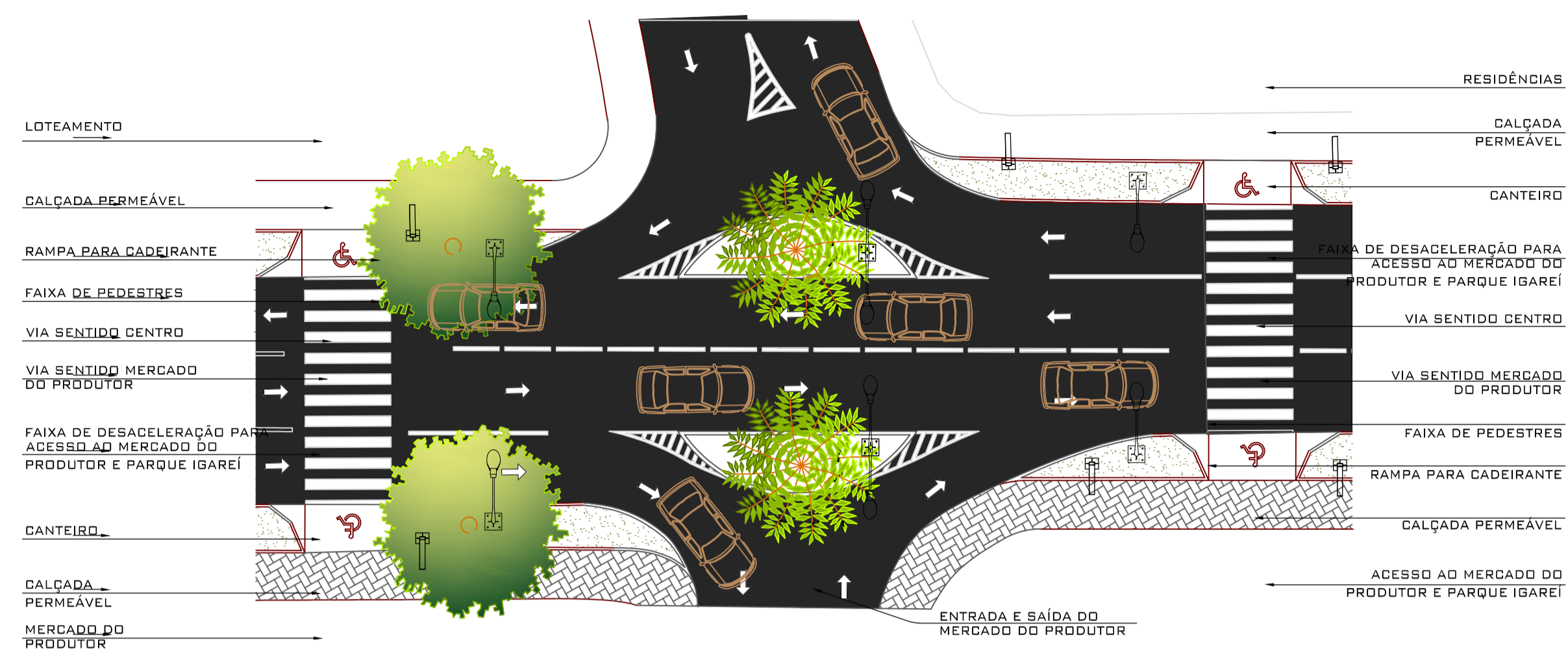
SEÇÃO ROTATÓRIA RUÁ ORMINDA VASCONCELOS ESC: 1/200
