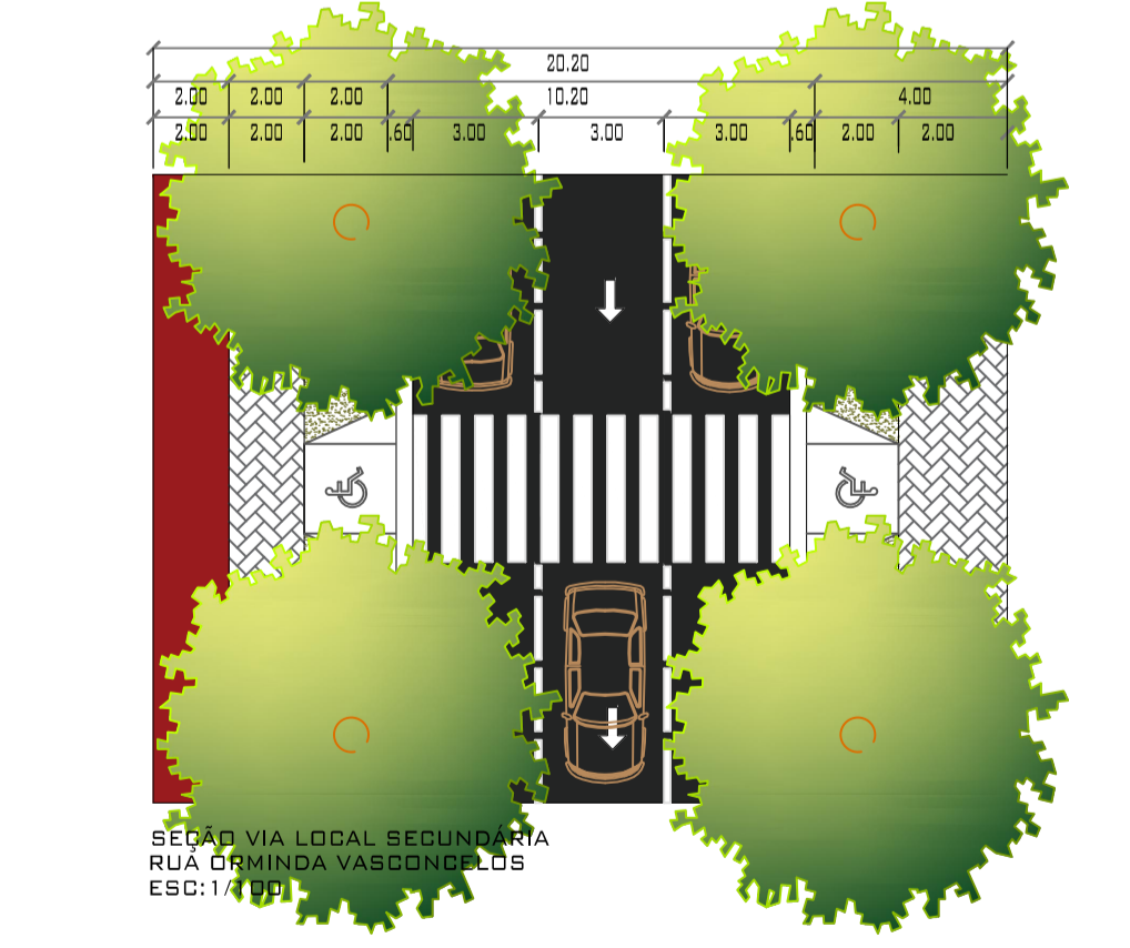
CORTE VIA LOCAL SECUNDÁRIA RUÁ ORMINDA VASCONCELOS ESC: 1/100
