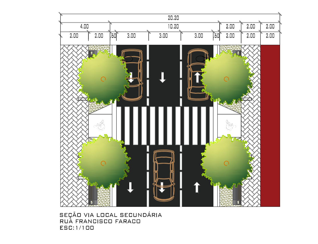
CORTE VIA LOCAL SECUNDÁRIA RUÁ FRANCISCO FARACO ESC: 1/100
