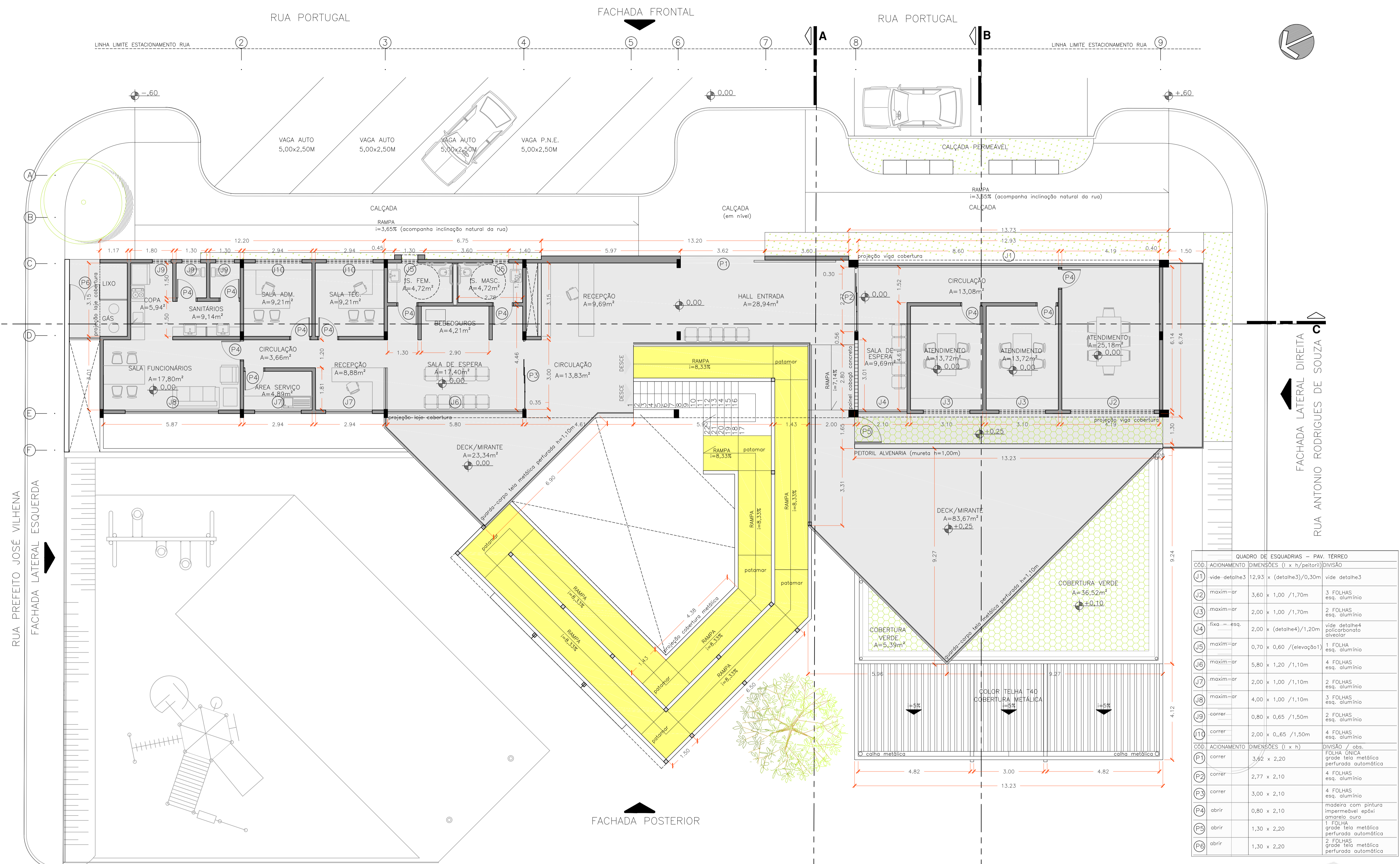
PLANTA TÉRREO escala 1:75
