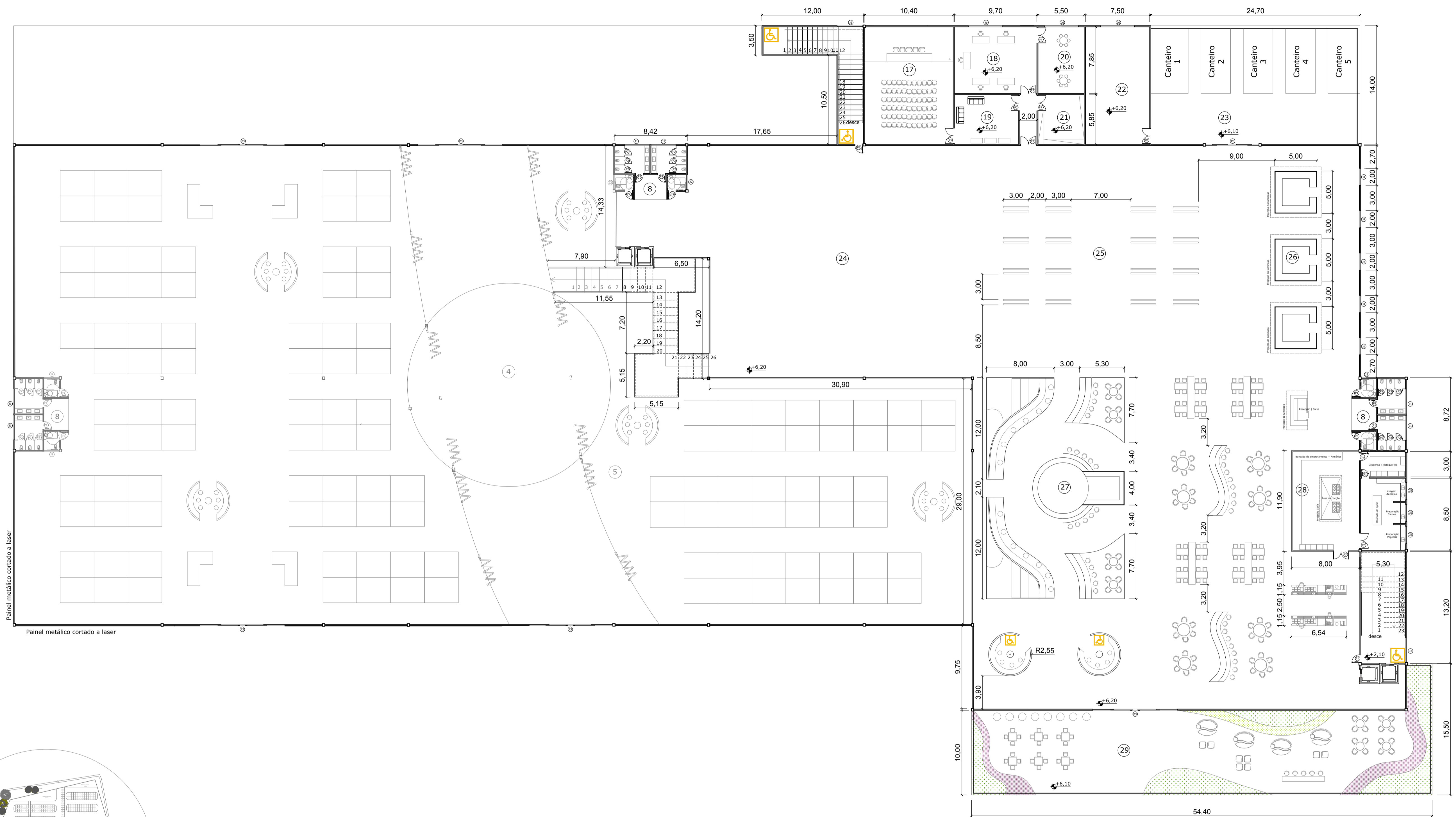
PLANTA MEZANINO Esc.: 1/250
