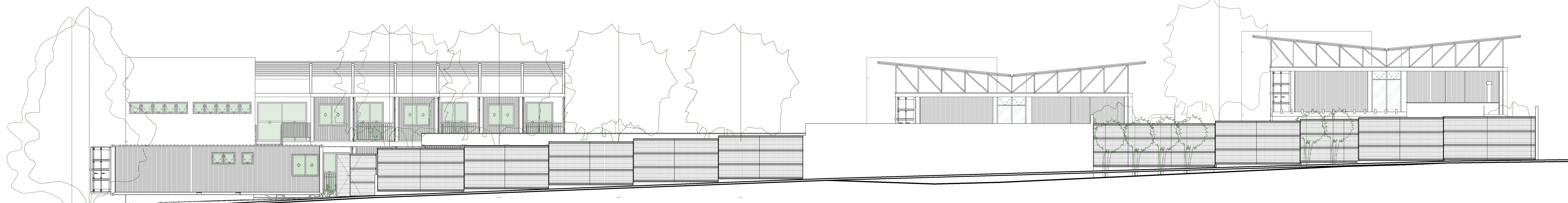
01 FACHADA 1:100
