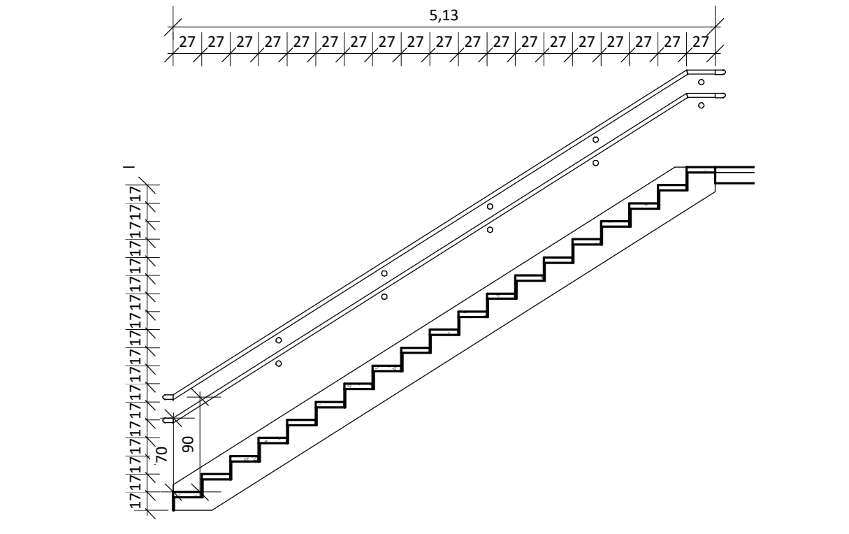
5 ESCADA 1:50
