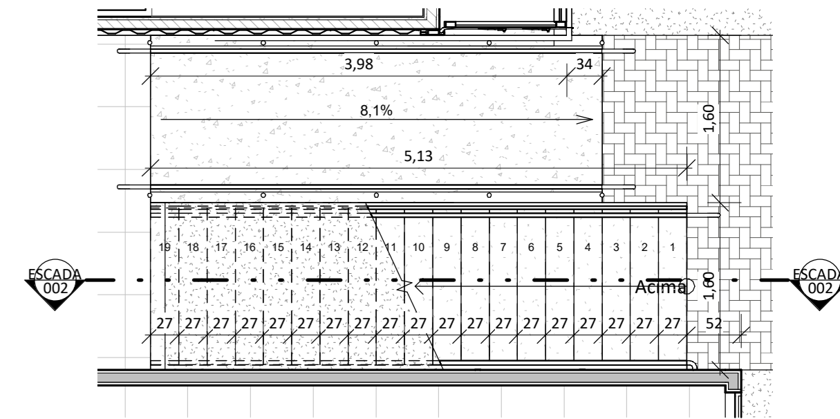
4 ESCADA 1:50
