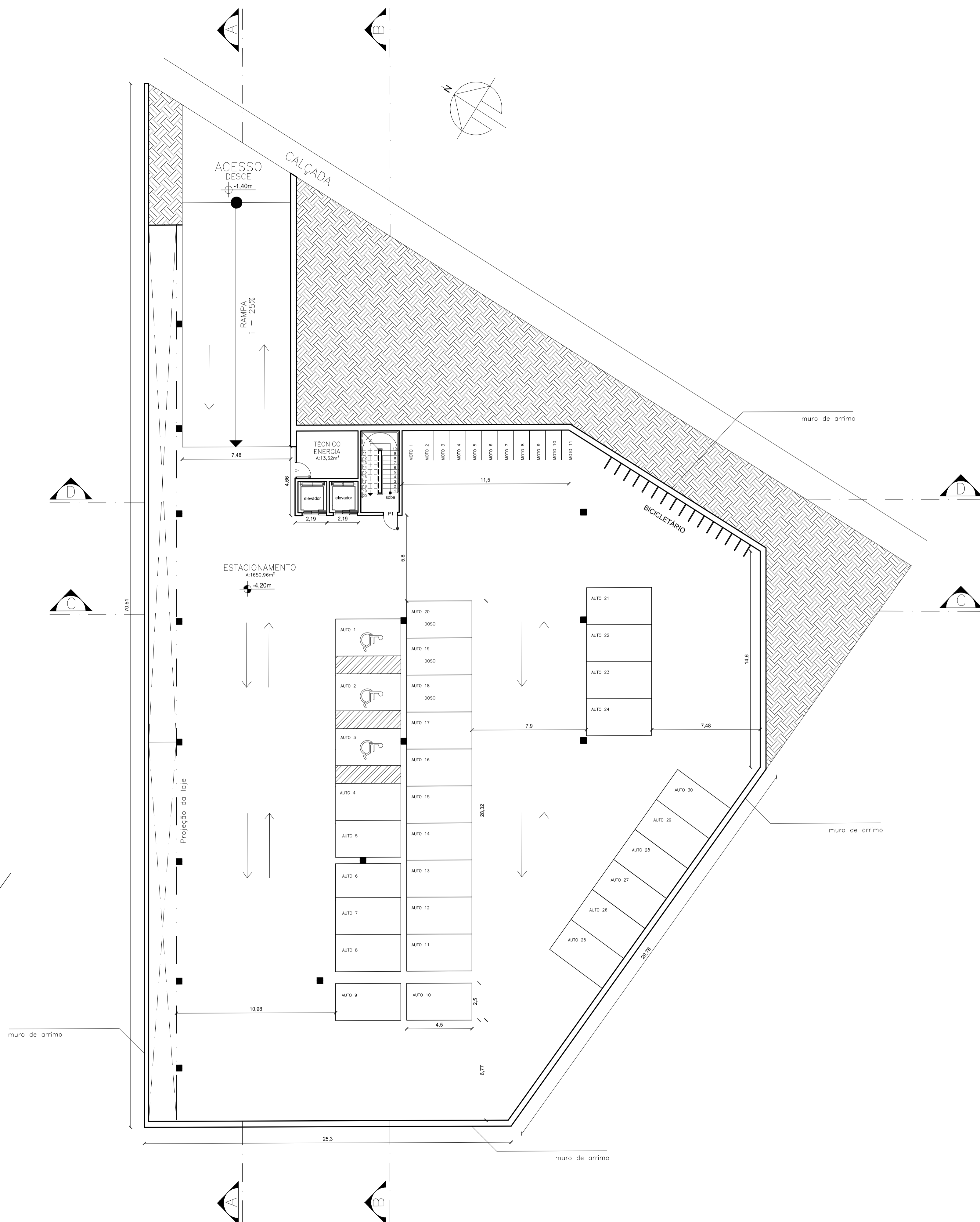
PLANTA ESTACIONAMENTO ESC: 1/125
