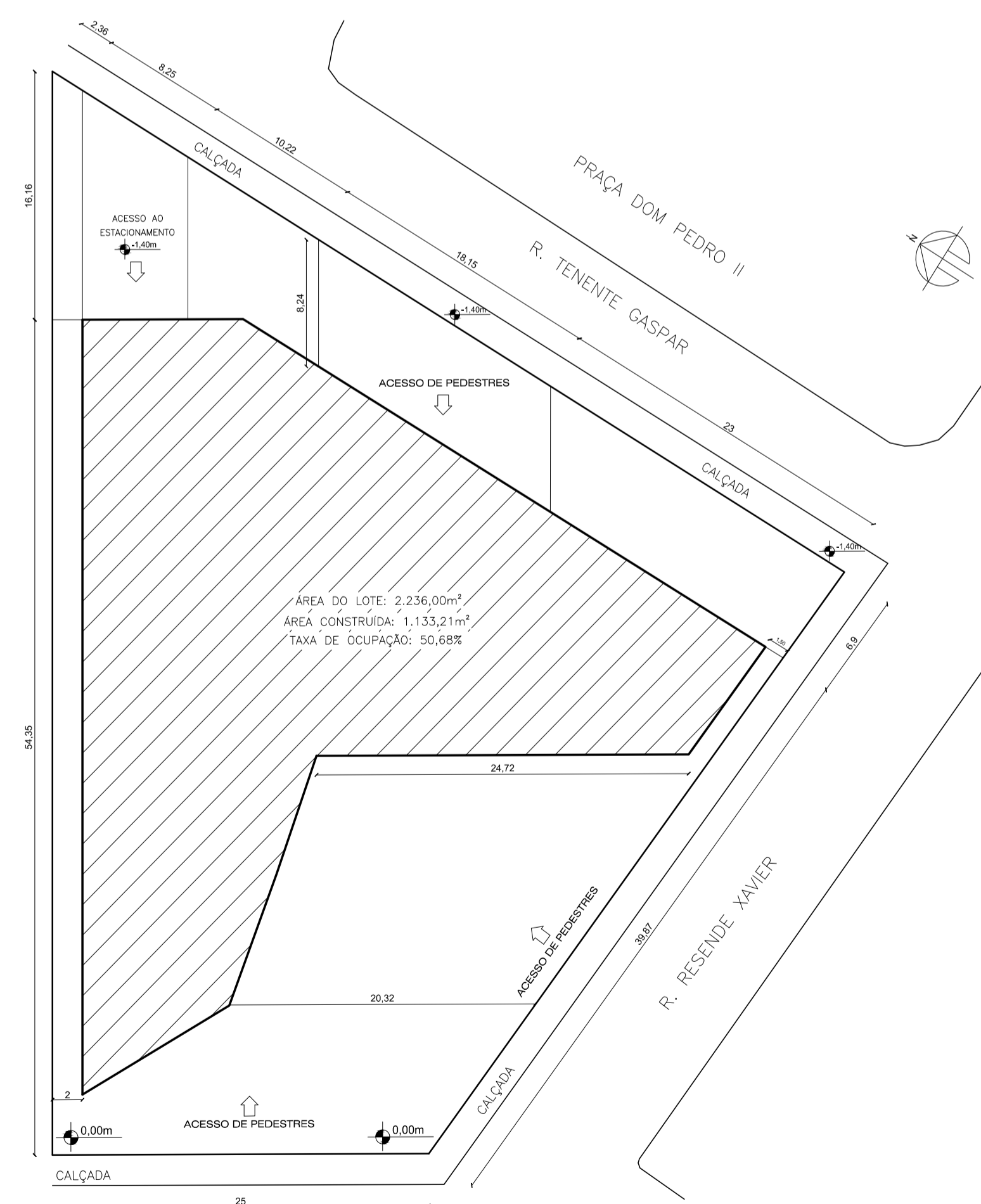
PLANTA DE IMPLANTAÇÃO ESC: 1/250
